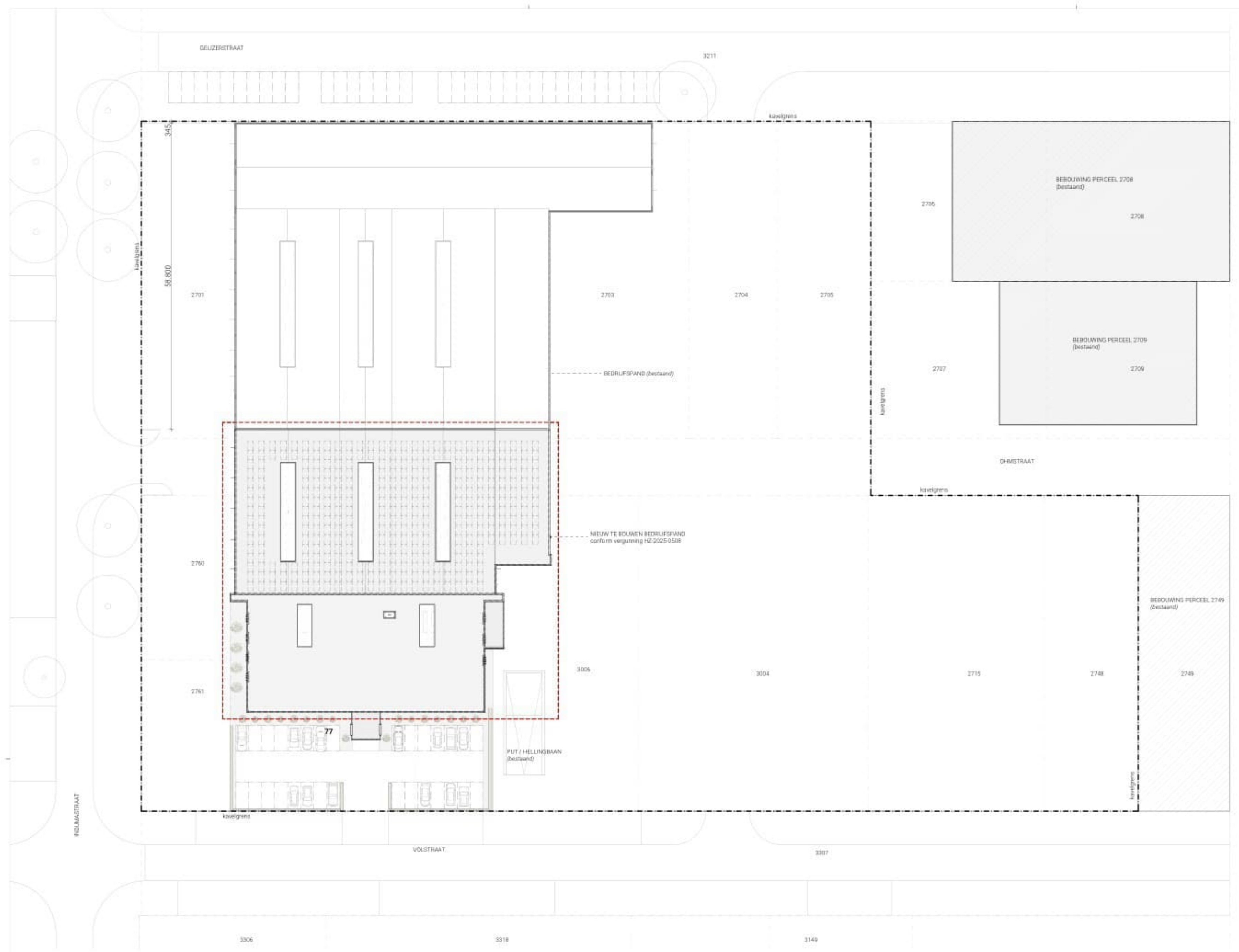
052 SITUATIE BESTAAND | 1:500
