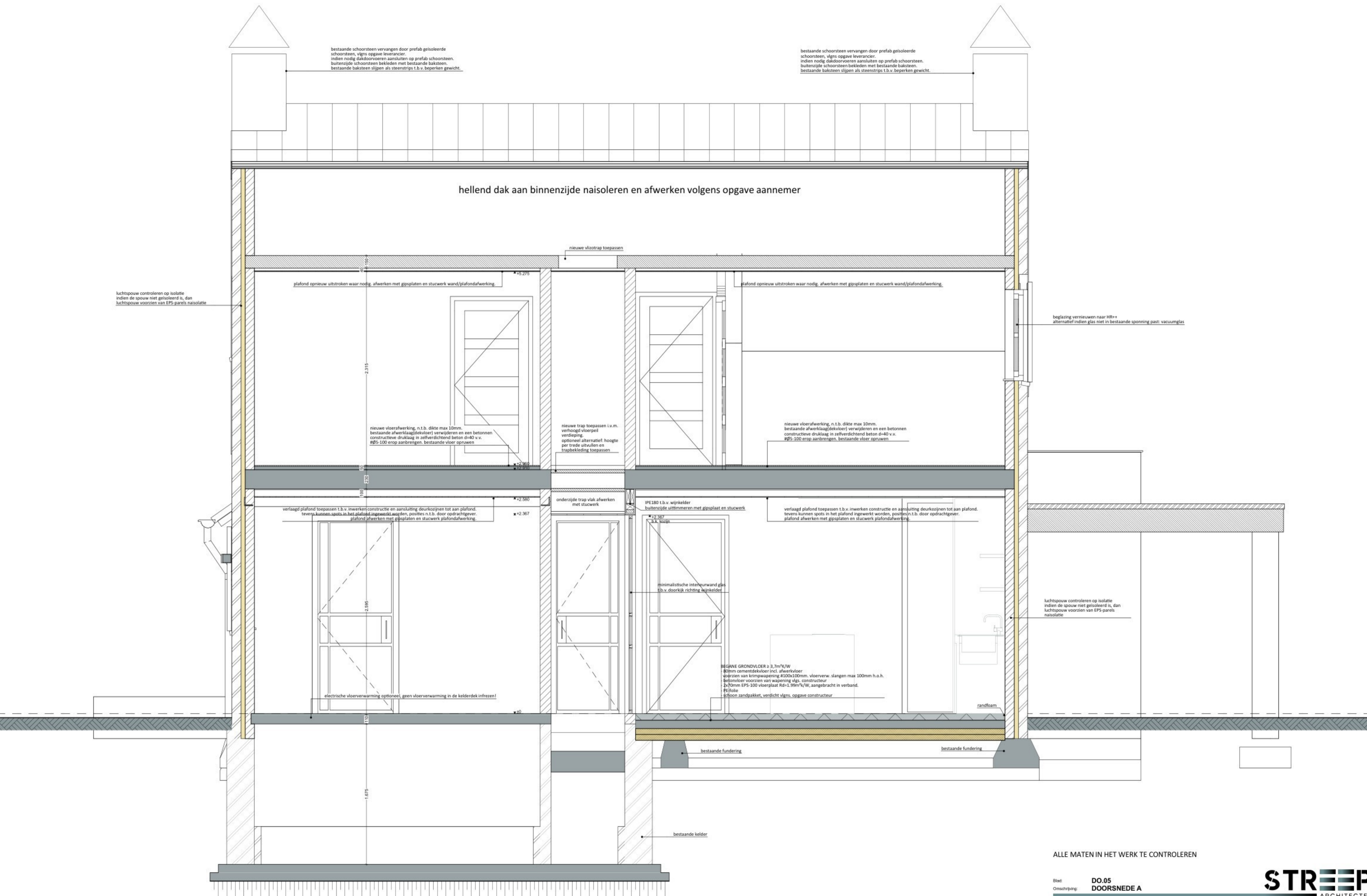
Doorsnede A-A
