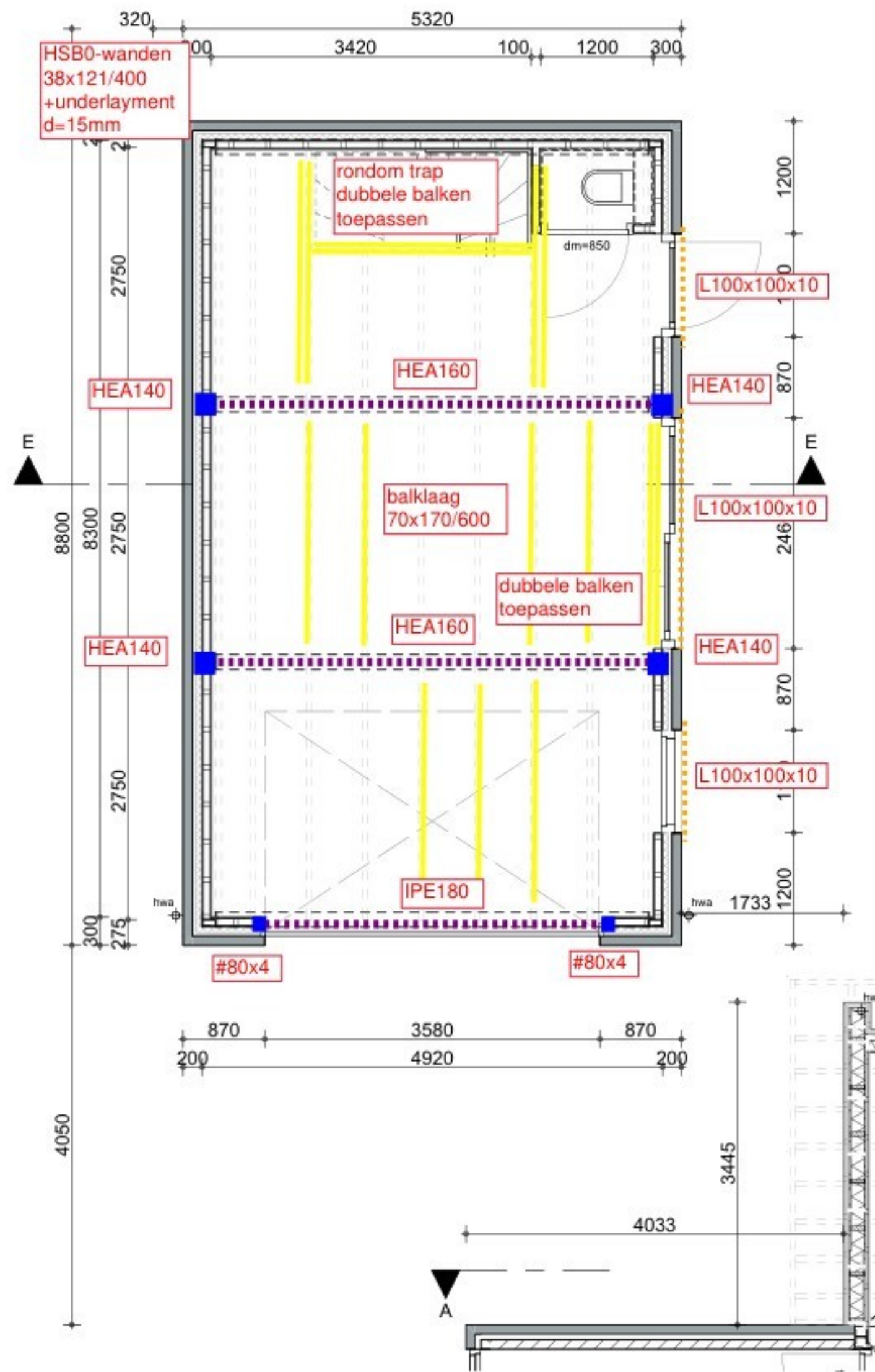
BEGANE GROND
