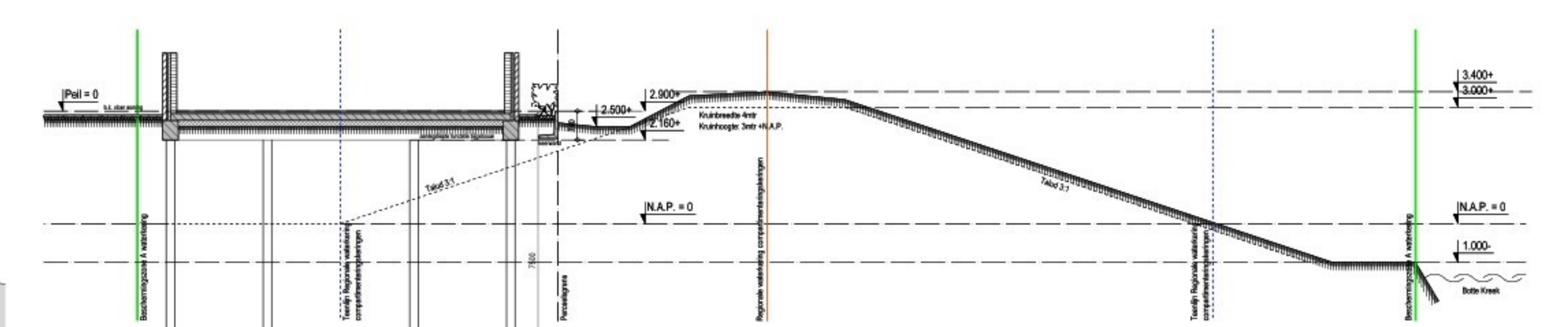
Doorsnede Regionale waterkering compartimenteringskeringen nieuwe toestand
