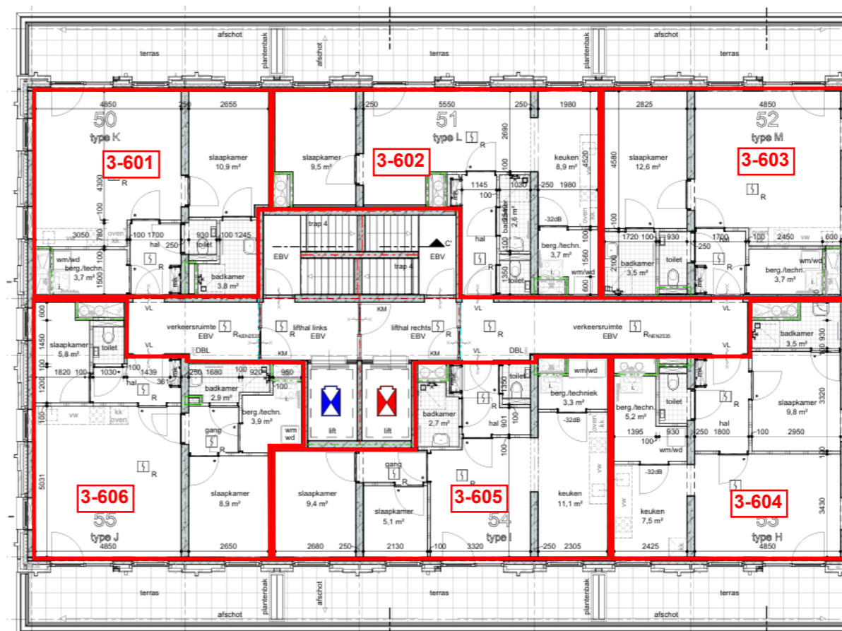
6e verdieping
