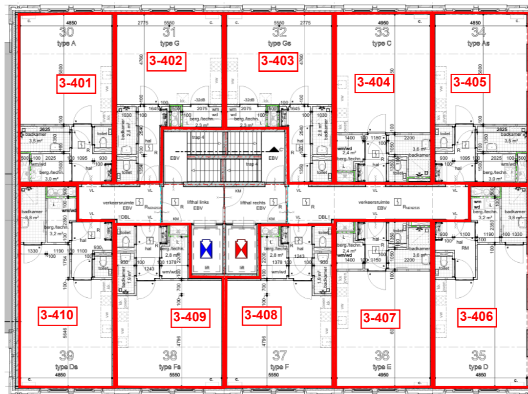
4e verdieping
