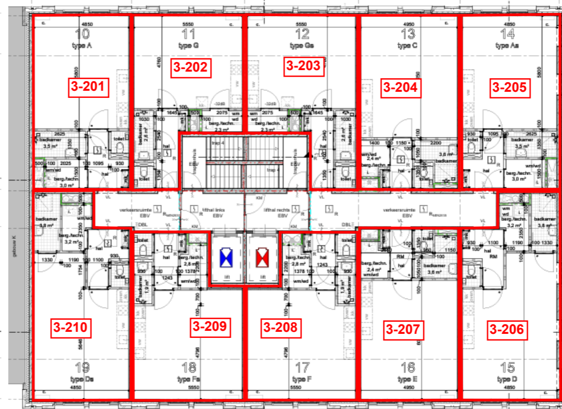
2e verdieping
