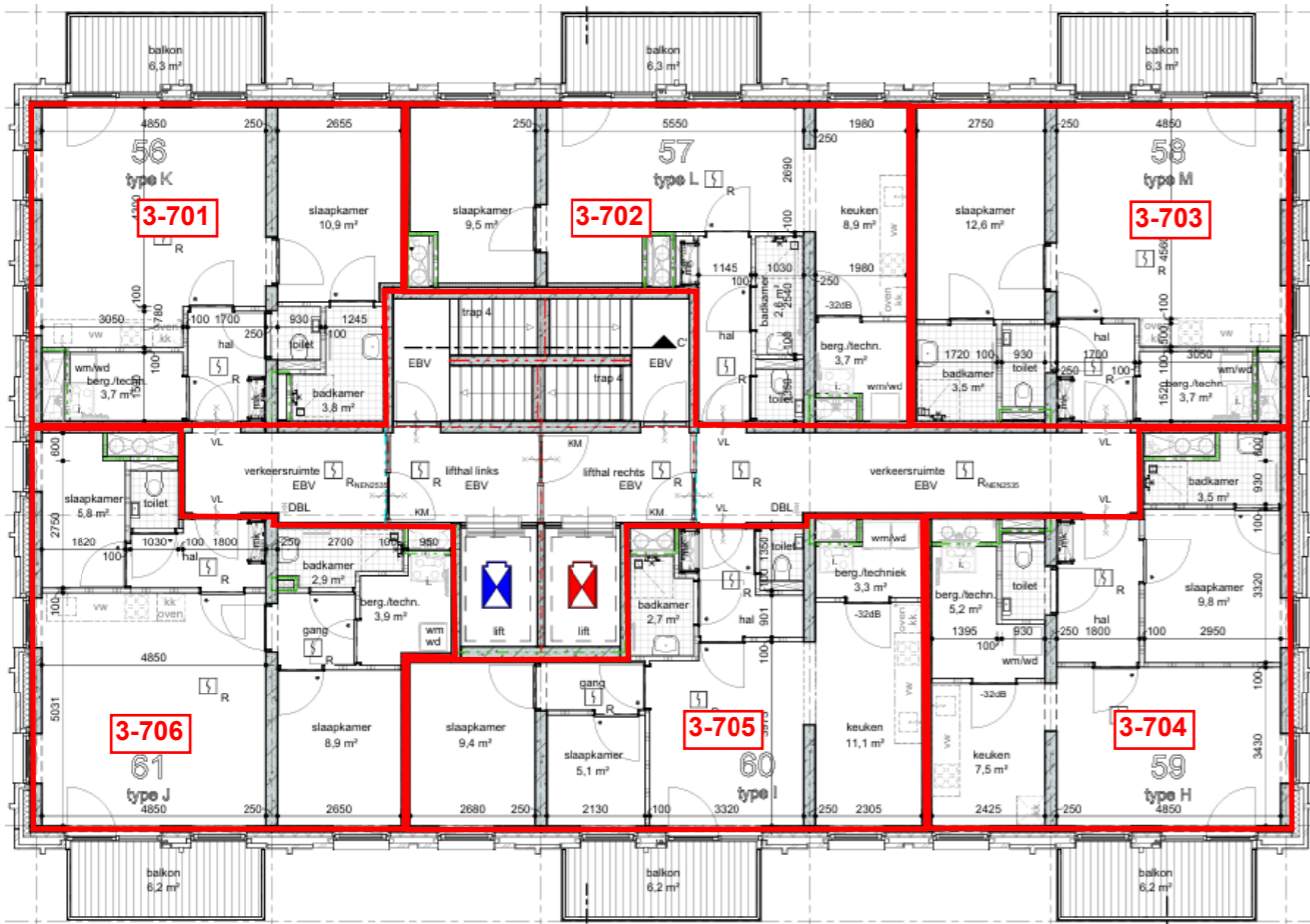
7e verdieping
