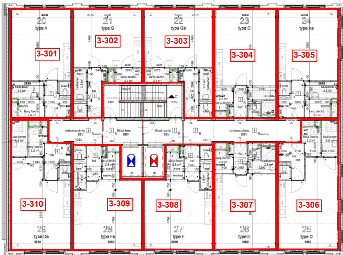
3e verdieping
