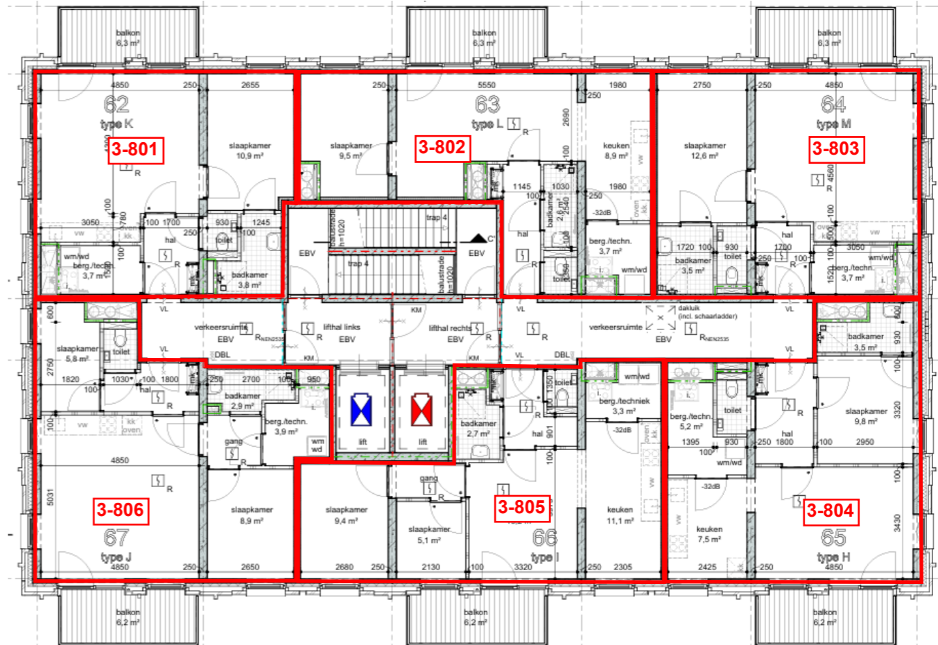
8e verdieping
