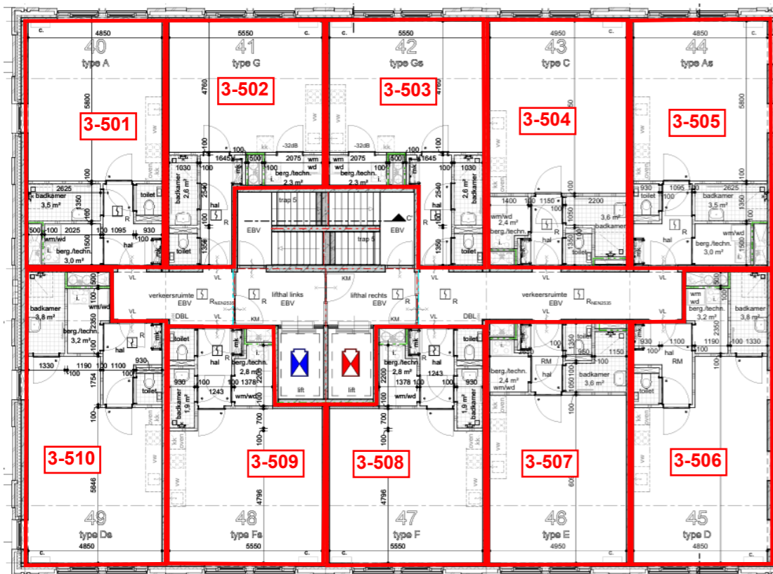
5e verdieping
