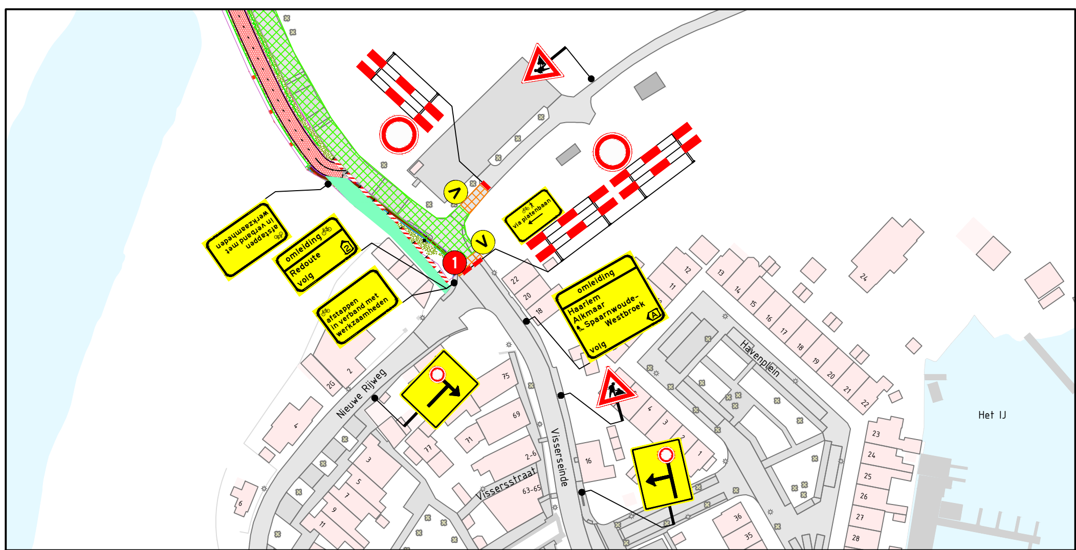
DETAIL 3 SCHAAL 1:1000
