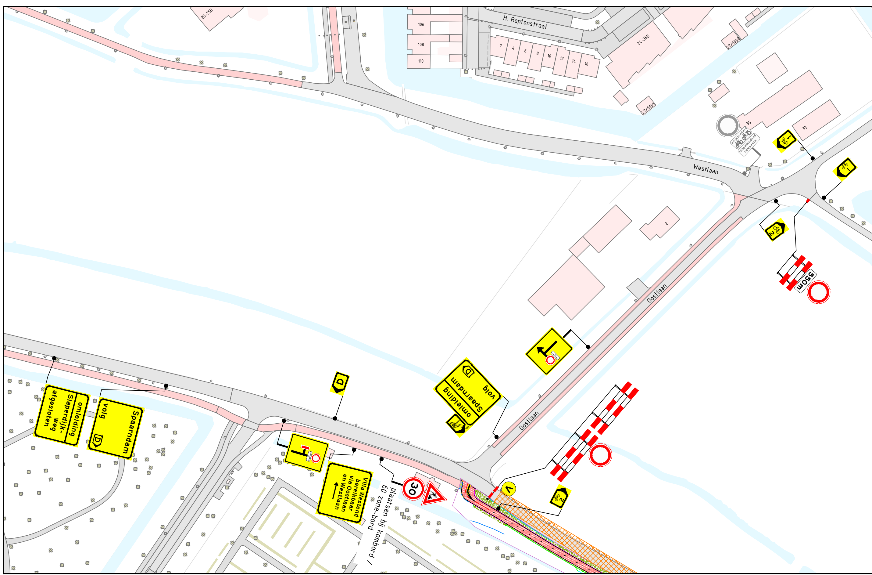
DETAIL 1 SCHAAL 1:1000
