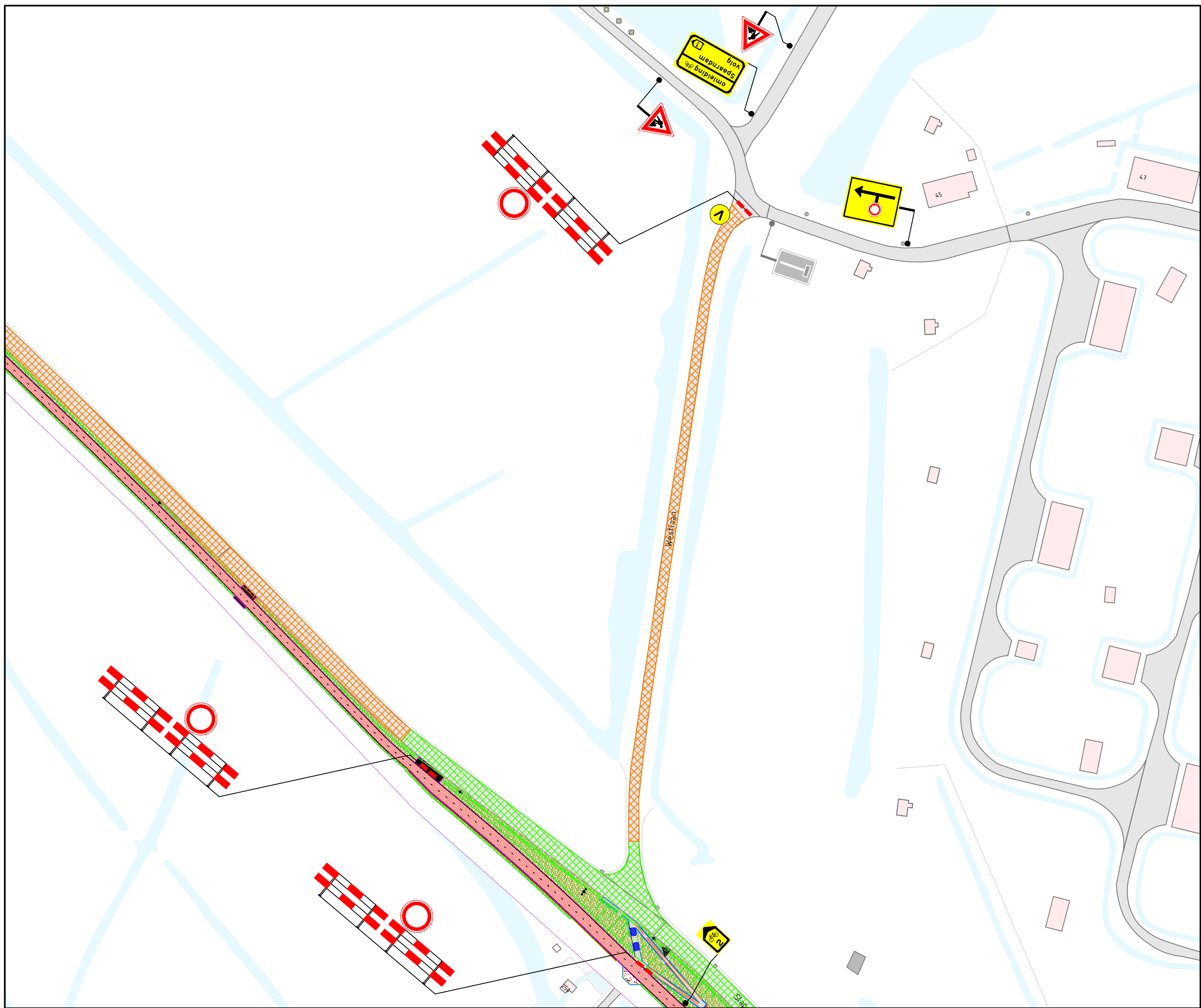
DETAIL 2 SCHAAL 1:1000
