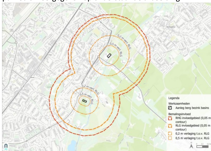
Figuur 2: Invloedsgebied bemaling bij hoge en lage grondwaterstand (RHG en RLG situatie), zie toelichting boven figuur voor uitgangspunten.
