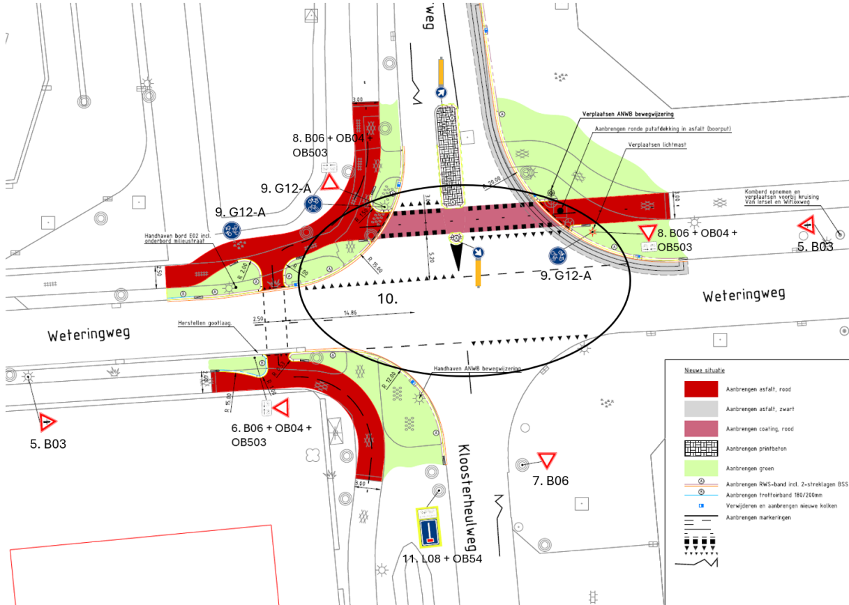
Tekening 2 het aanbrengen van de nieuwe situatie
