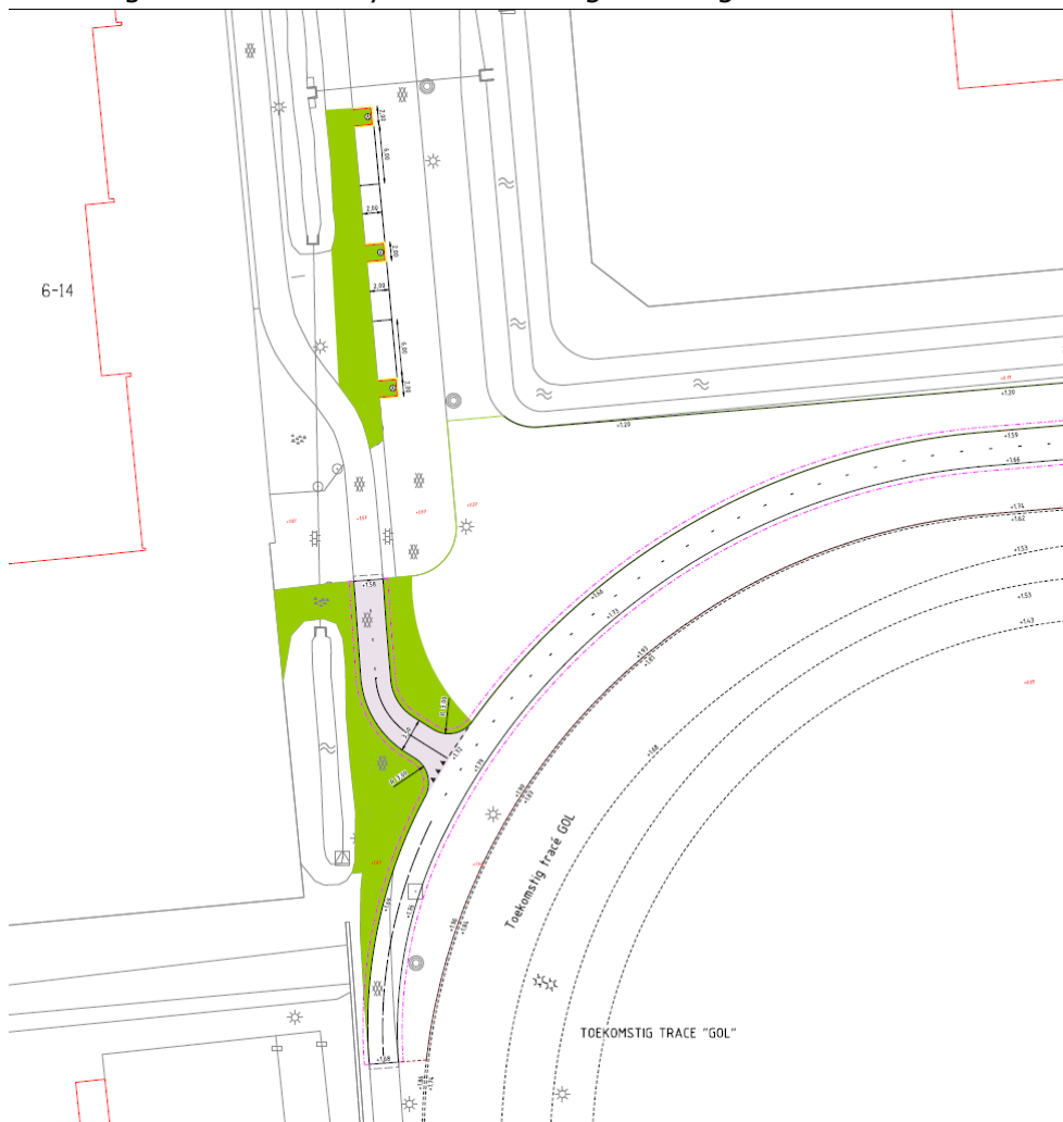
Tekening 4: De nieuwe fysieke afsluiting ter hoogte van nummer 6.
