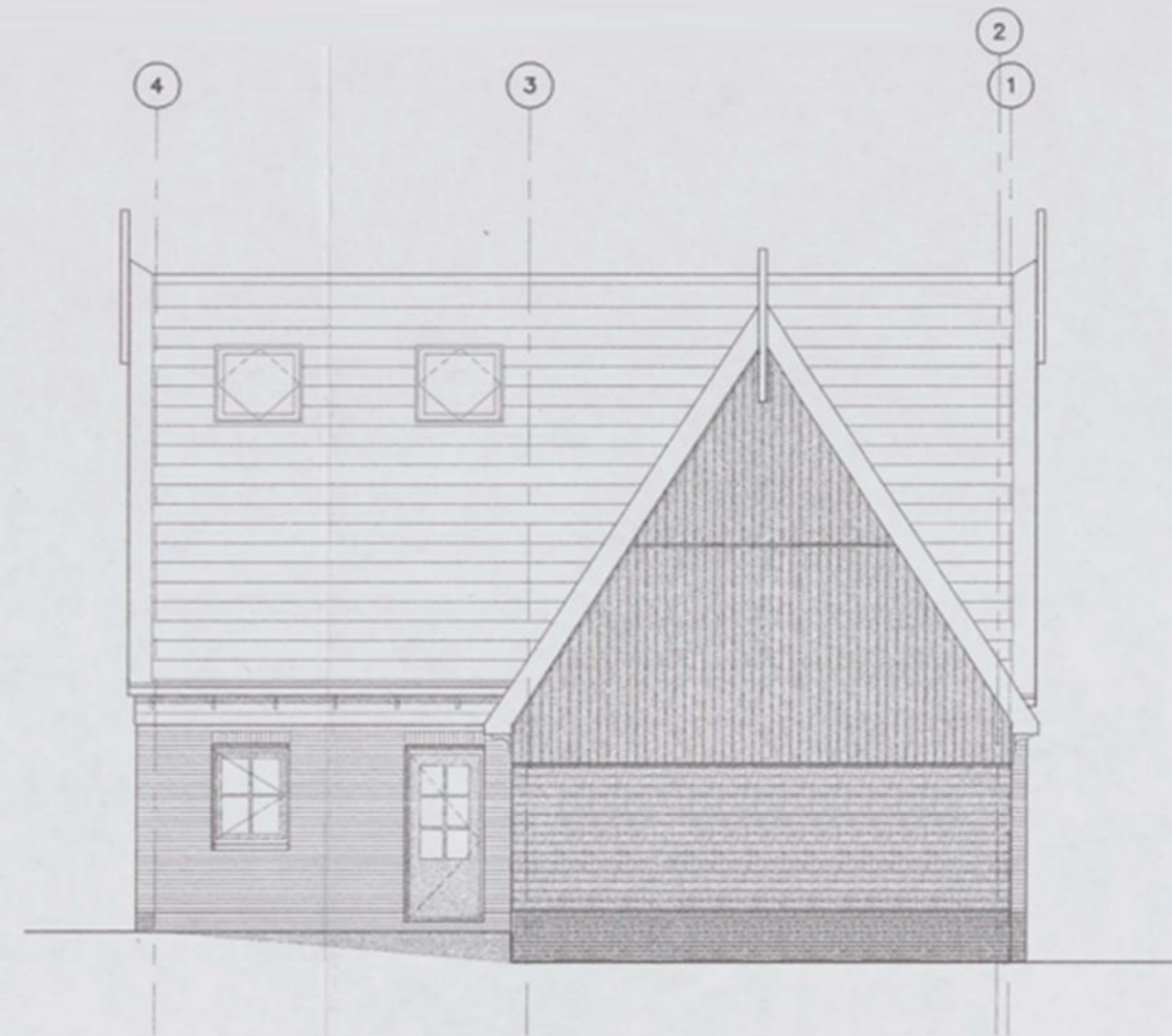
Rechter zijgevel nieuwe situatie
