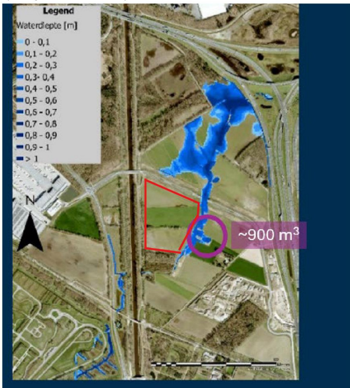
Figuur 2-1 Berekend maximaal overstromingsbeeld T=10 referentie situatie
