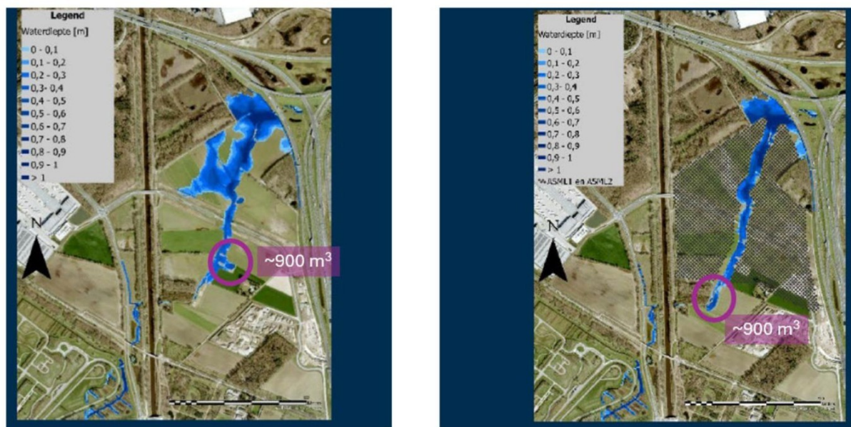
Figuur 2-1 Berekend maximaal overstromingsbeeld T=10 referentie situatie (links) en basisscenario BIC (rechts)
