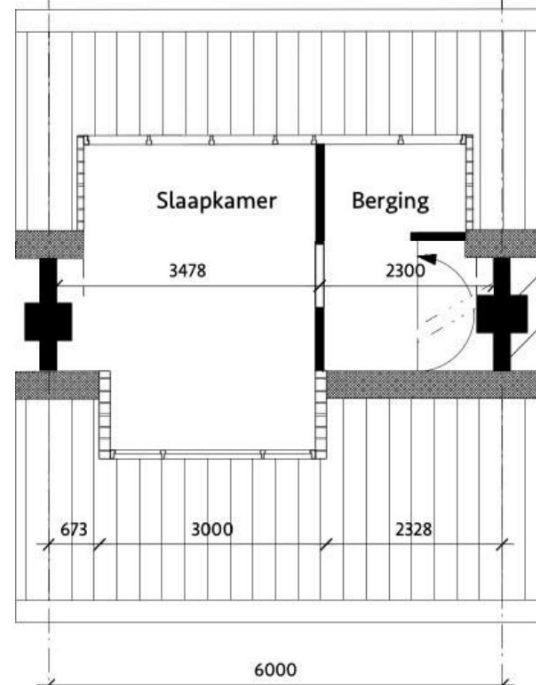
2e Verdieping - gewijzigd
