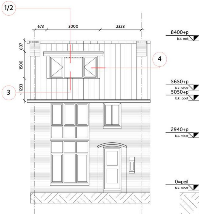
Voorgevel - gewijzigd
