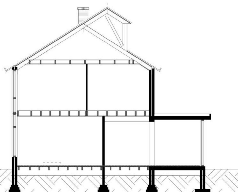
Doorsnede - bestaand
