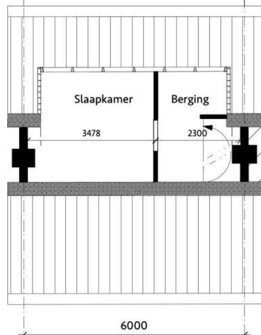
2e Verdieping - bestaand
