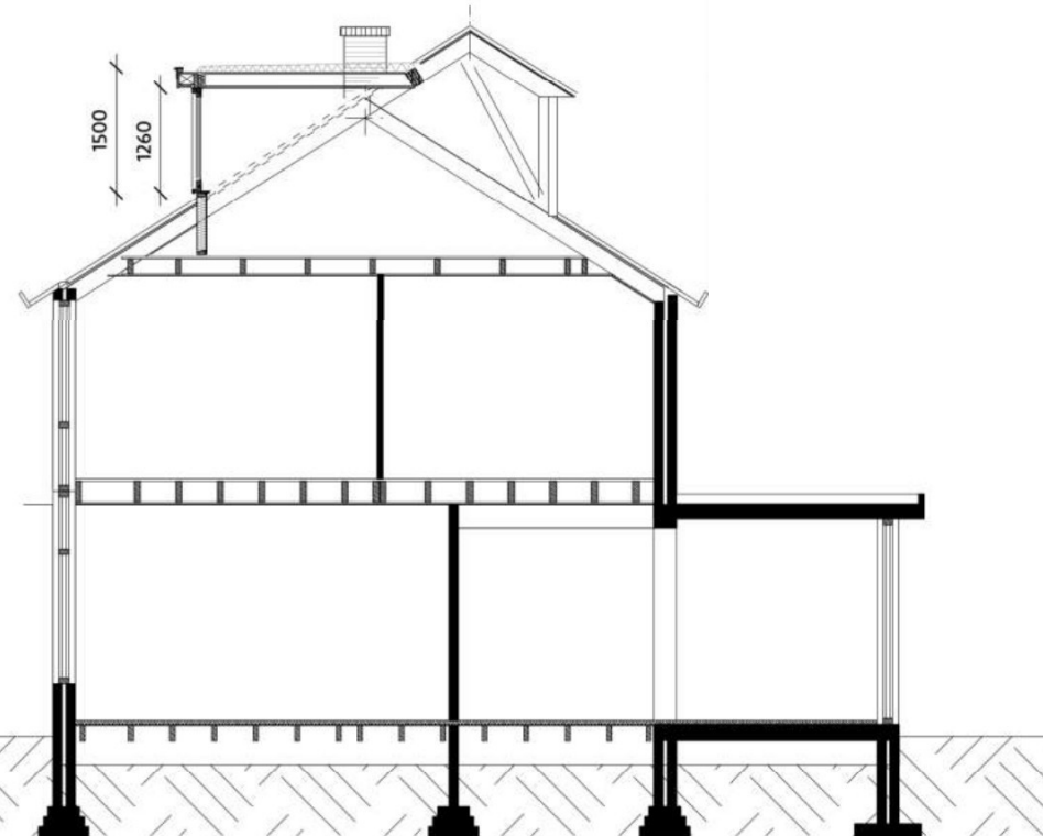
Doorsnede - gewijzigd
