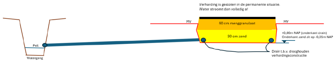
Figuur 3.3 Schematische toelichting werking systeem 1 eindfase
