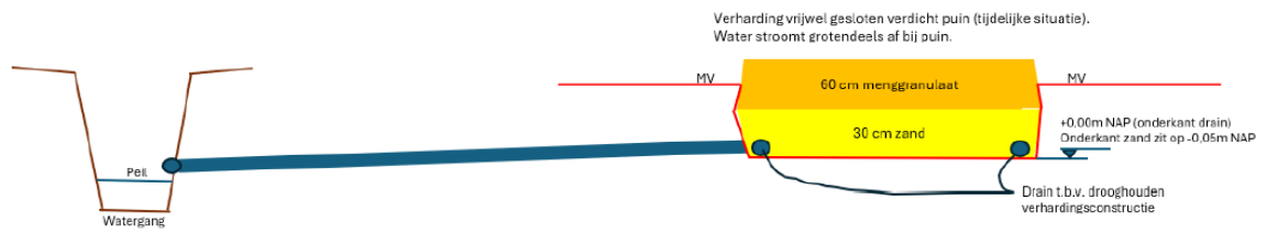
Figuur 3.2 Schematische toelichting werking systeem 1 tijdelijke fase
