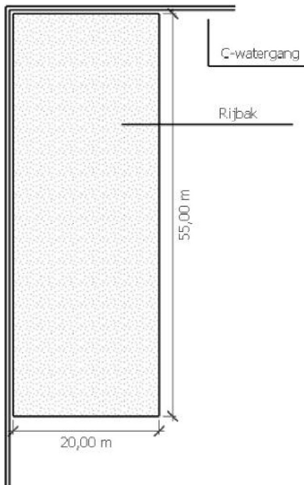
Figuur 4: Bovenaanzicht rijbak, in de tekening bovenaan en links van de rijbak loopt de c-watergang
