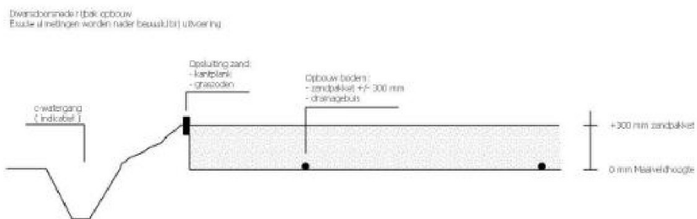
Figuur 5: Dwarsdoorsnede rijbak opbouw (exacte afmetingen worden nader bepaald tijdens uitvoering)
