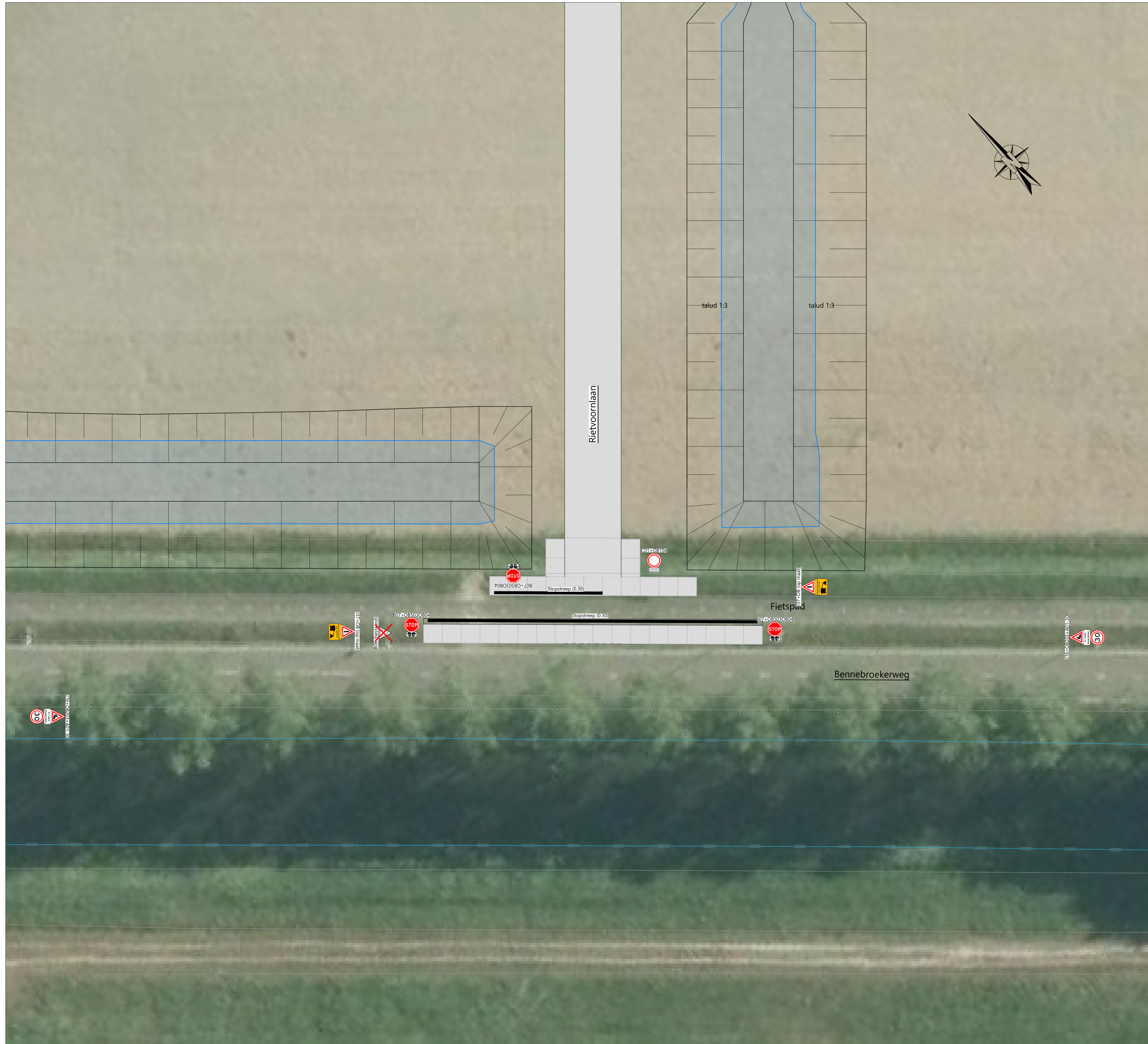
Situatie aansluiting Bennebroekerweg Schaal 1:200
