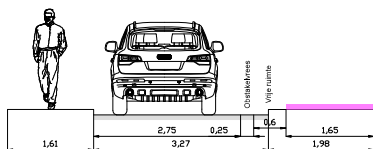
Dwarsprofiel A Schaal: 1:100
