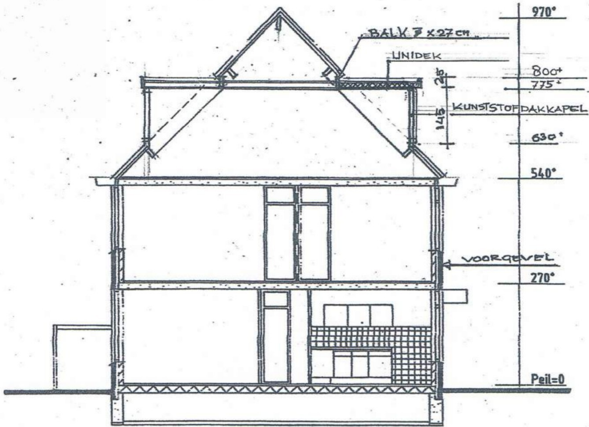
DOORSNEDE NIEUW
