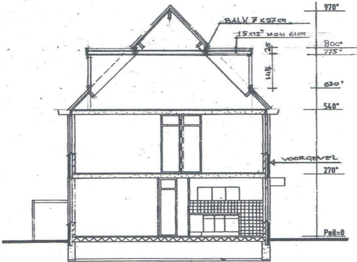
DOORSNEDE BESTAAND SCHAAAL 1:100
