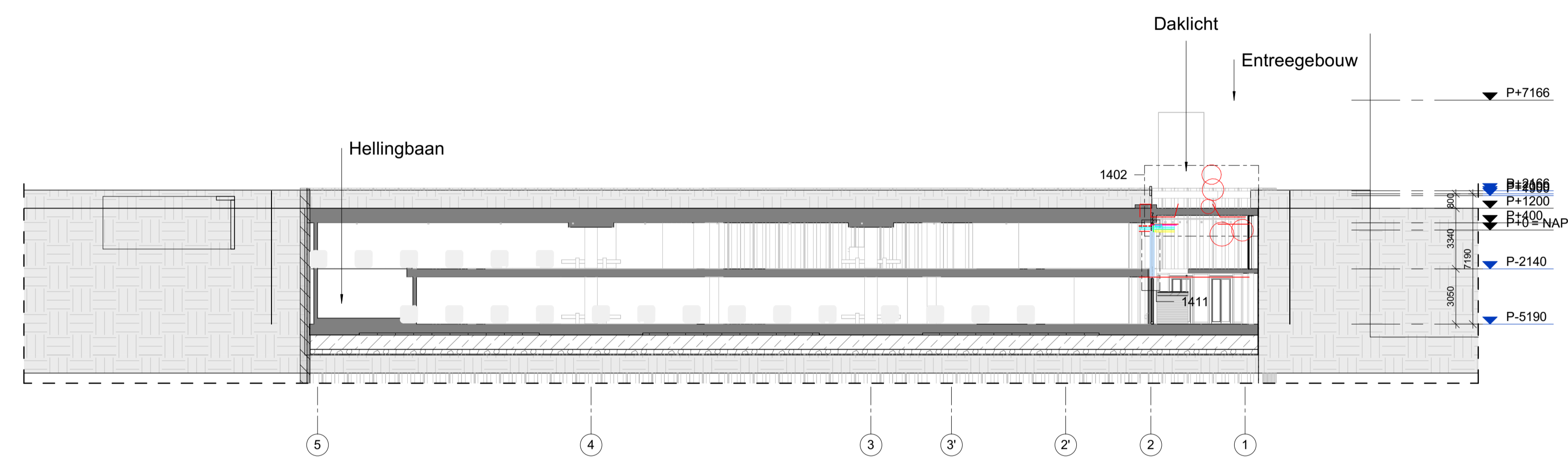
DS B1 1:200
