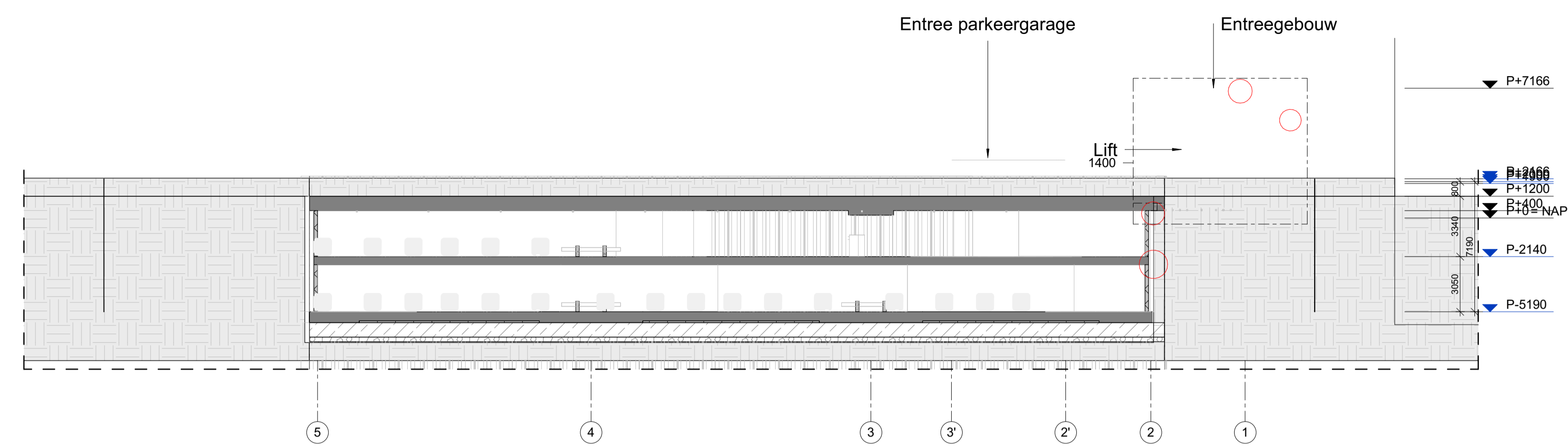
DS B 1:200
