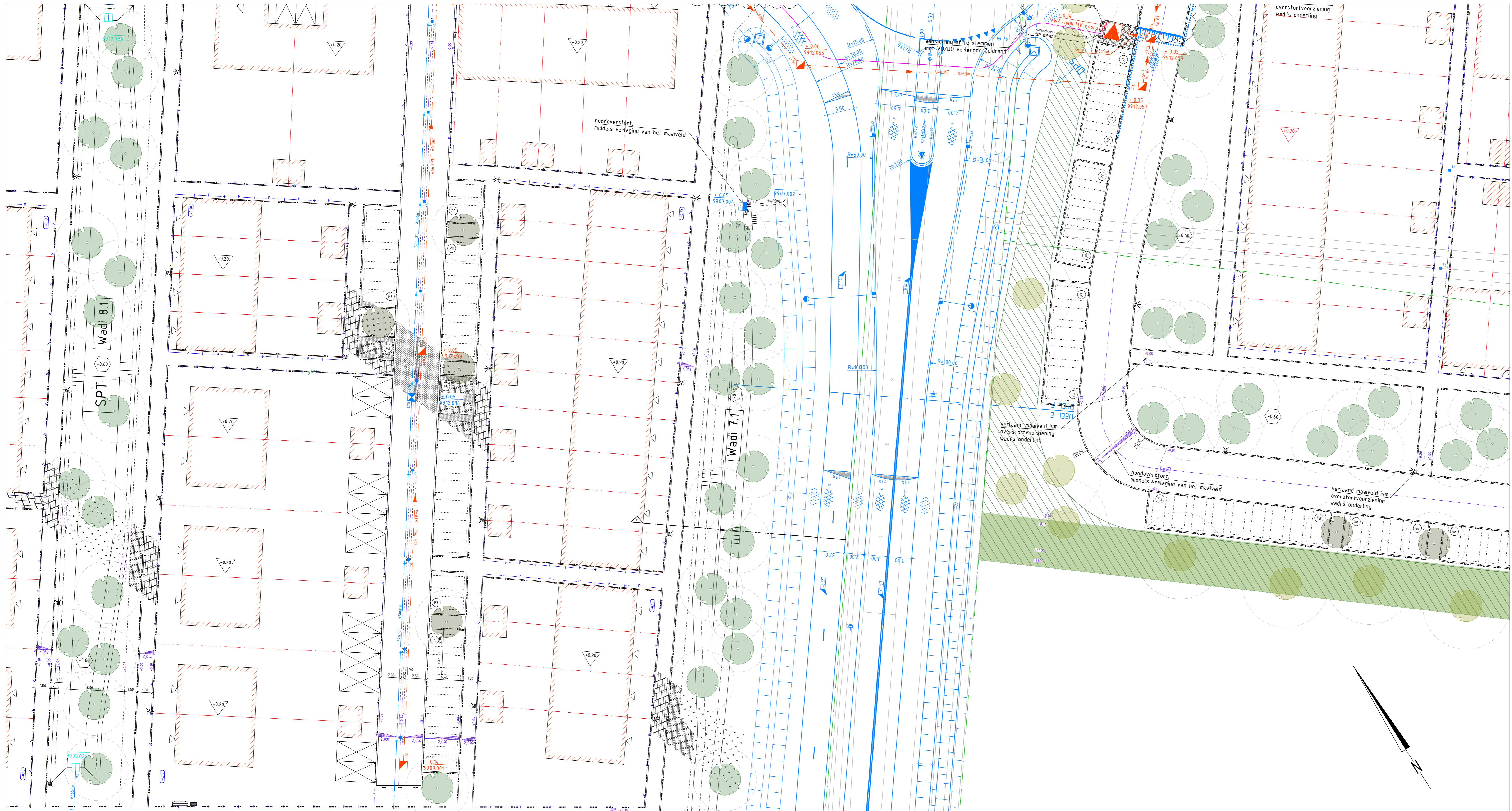
Situatie nabij profiel 10 Schaal 1:200
