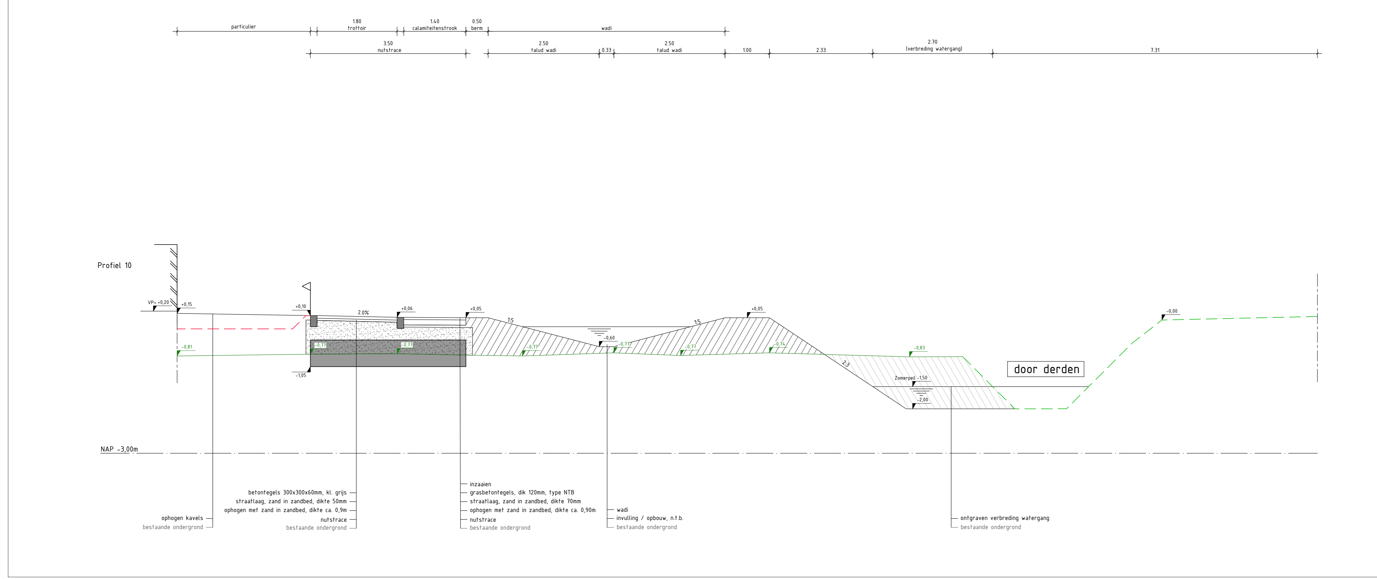
Profiel 10 Schaal 1:50
