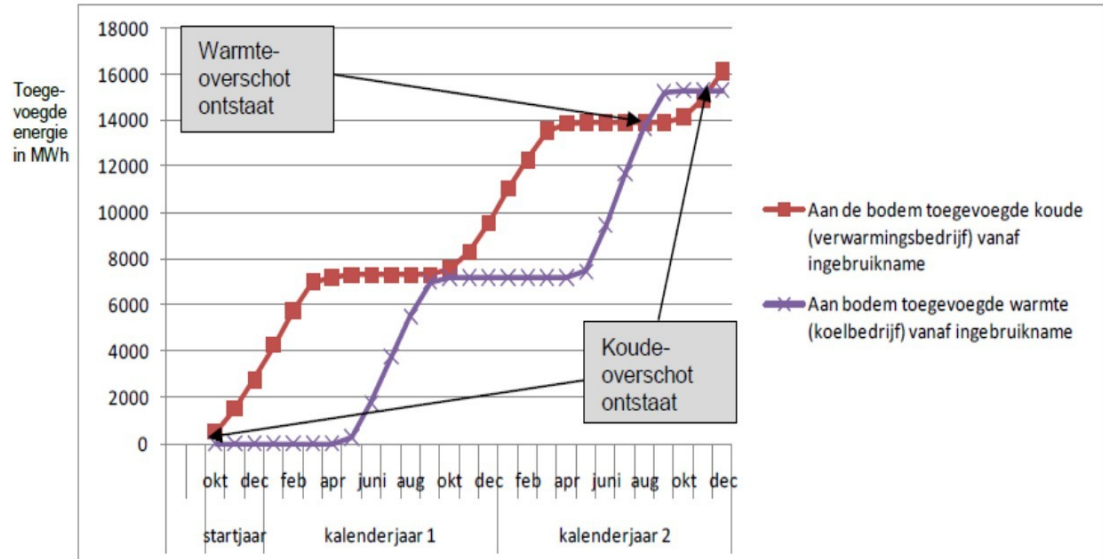
Figuur 1. Illustratie weergave van aan de bodem toegevoegde koude en warmte tijdens de gebruiksfase.
