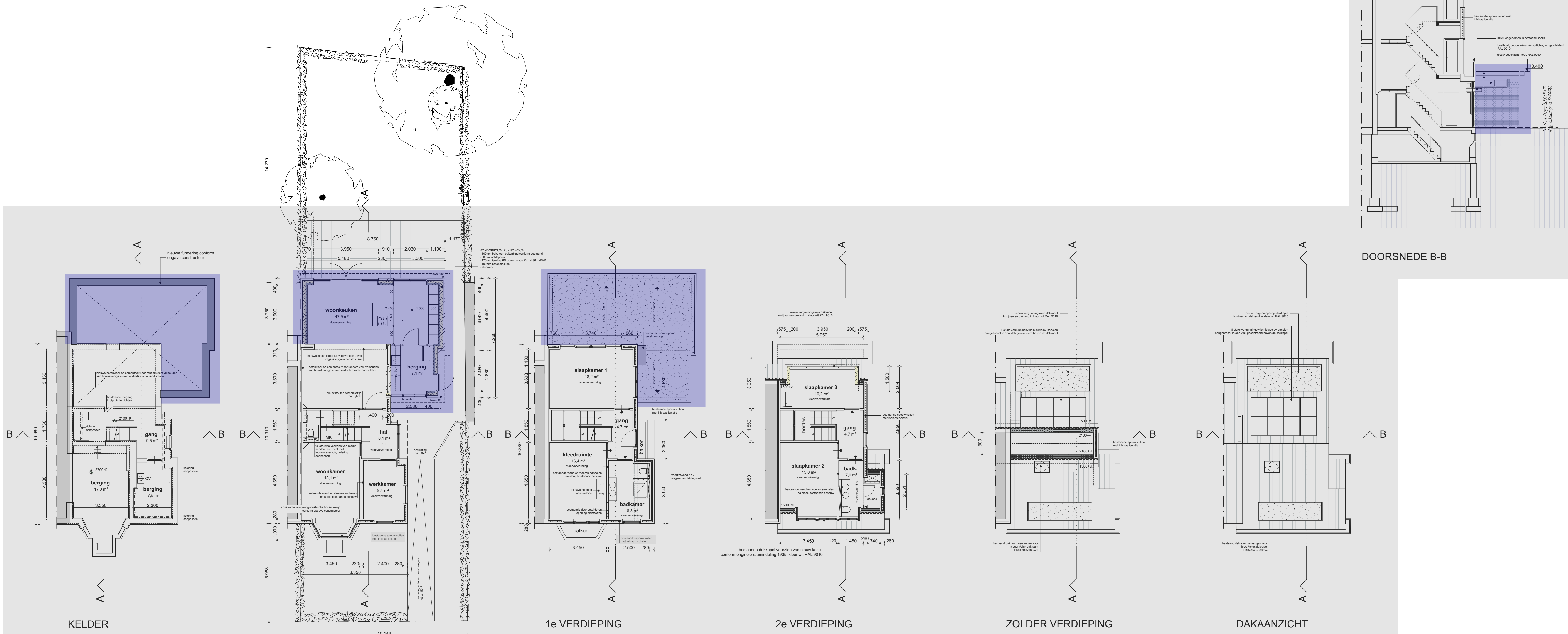
BEGANE GROND
