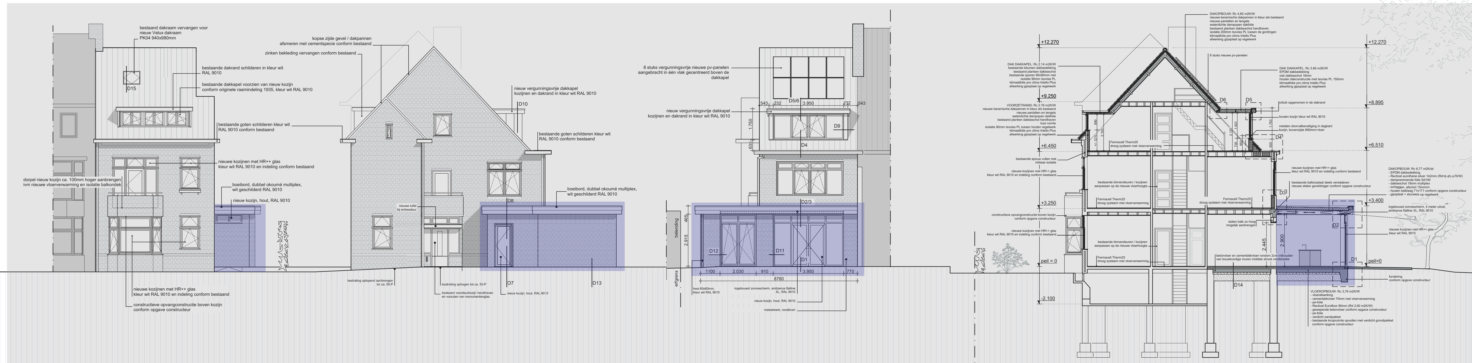
VORGEVEL
