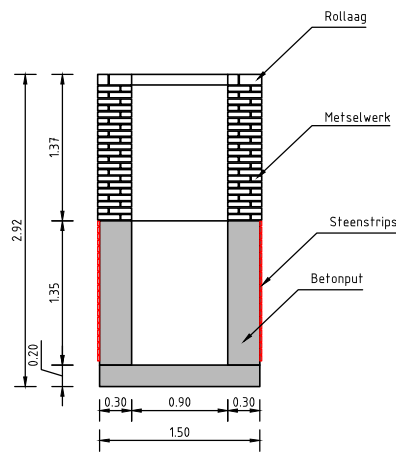
Principe 2: Prefab betonput met steenstrips en metselwerk
