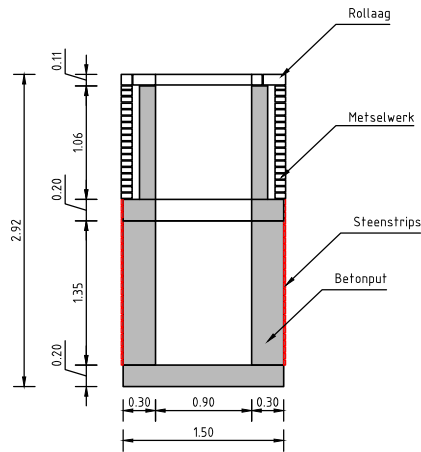
Principe 1: Prefab betonput met steenstrips en deels metselwerk
