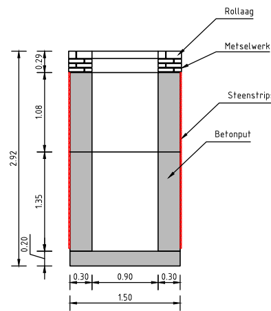
Principe 3: Prefab betonput met alleen bovenste deel metselwerk en overige delen in steenstrips
