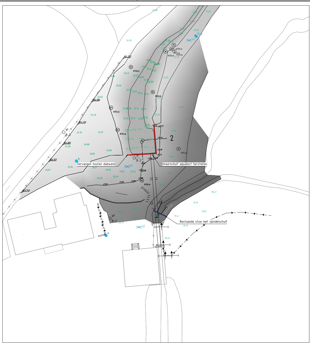
Situatie Schaal 1:200
