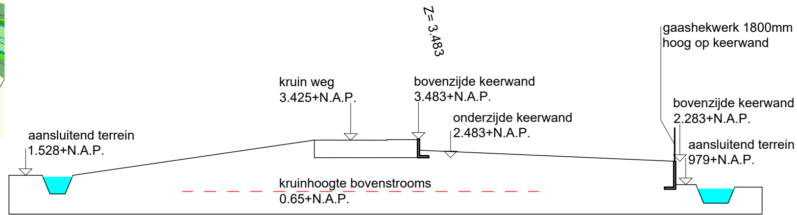
principe doorsnede dijklichaam regionale waterkering langs regionale rivier
