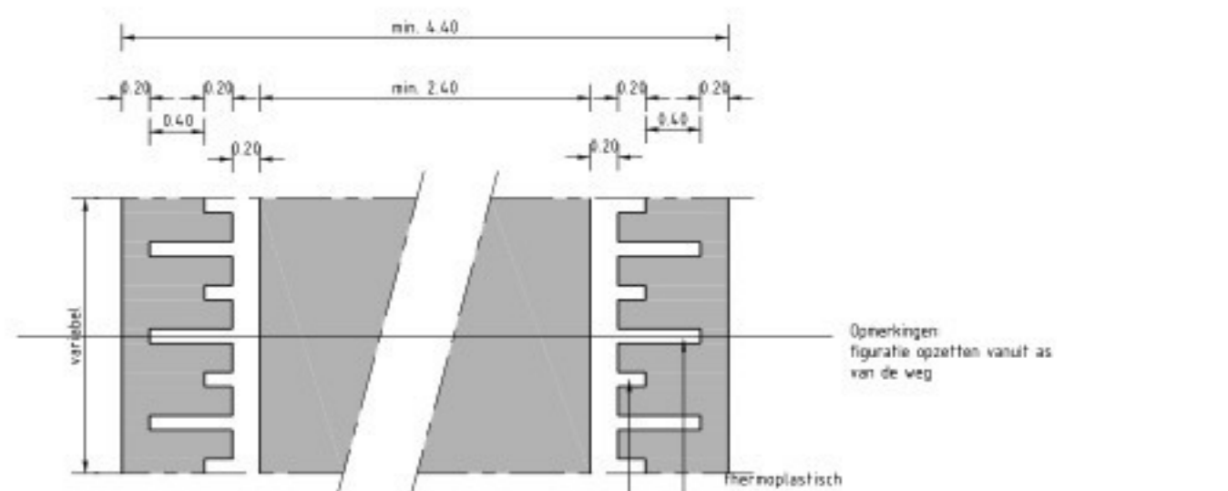
Dwarsdoorsnede Plateau van BSS (30 km/uur)
