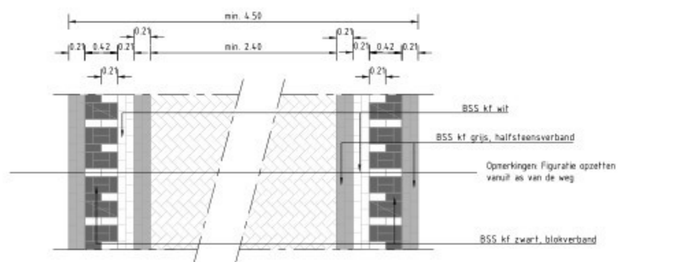
Dwarsdoorsnede Plateau van BSS (30 km/uur)
