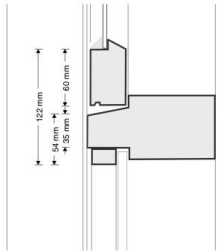
D1 tussendetail bestaand
