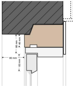
D1 bovendetail bestaand
