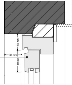
D1 bovendetail nieuw
