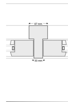
D3 tussendetail nieuw
