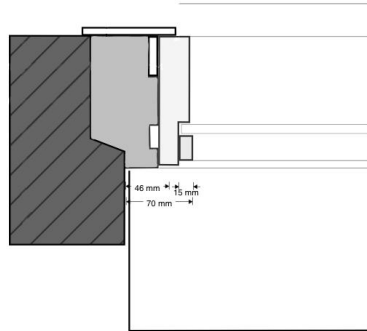
D3 zijdetail bestaand
