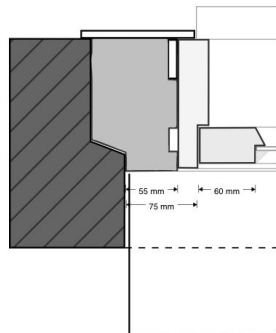
D2 zijdetail bestaand
