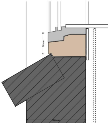
Kozijn bestaand
