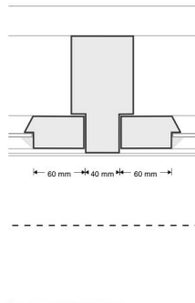
D3 tussendetail bestaand
