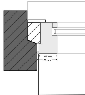
D3 zijdetail nieuw
