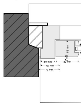
D2 zijdetail nieuw
