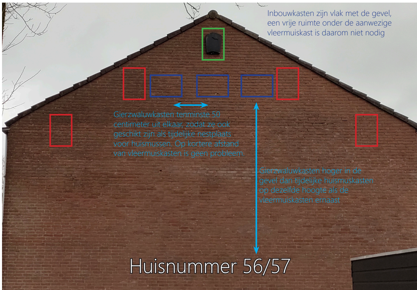
Afbeelding 5: Foto van de kopgevel van De Valkhof, huisnummer 73, indicatief voor huisnummers 56/57, met daarop aangegeven op welke wijze nieuwe voorzieningen ingepast zullen worden. In groen de huidige aanwezige tijdelijke vleermuiskast, in rood de nieuw in te bouwen vleermuiskasten en in donkerblauw de nieuw in te bouwen gierzwaluwkasten.
