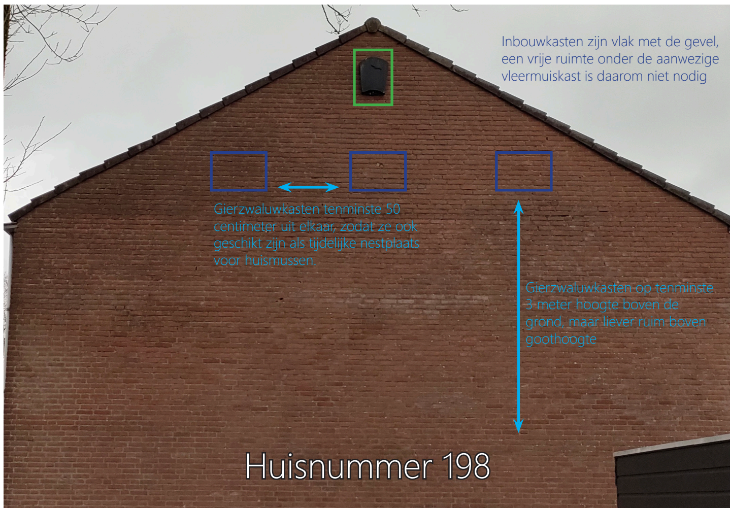
Afbeelding 14: Foto van de kopgevel van De Valkhof, huisnummer 73, indicatief voor huisnummers 198, met daarop aangegeven op welke wijze nieuwe voorzieningen ingepast zullen worden. In groen de huidige aanwezige tijdelijke vleermuiskast en in donkerblauw de nieuw in te bouwen gierzwaluwkasten.
