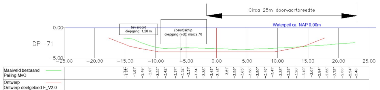
Figuur 2 Principedwarsprofiel met baggerponton en binnenvaartschip CEMT-IV
