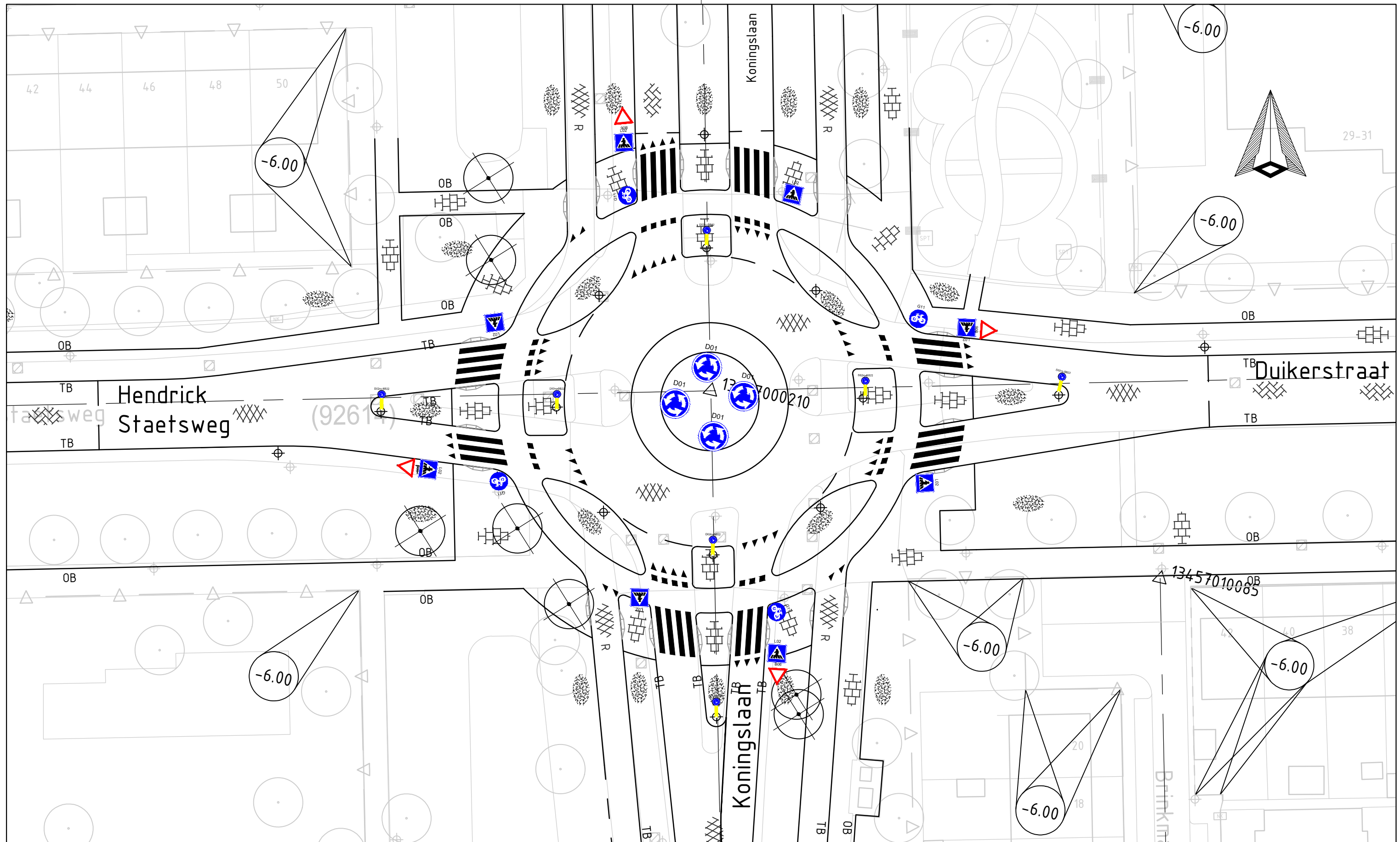
Kruispunt Hendrik Staetsweg - Duikerstraat - Koningslaan rotonde Tekening voor verkeersbesluit
