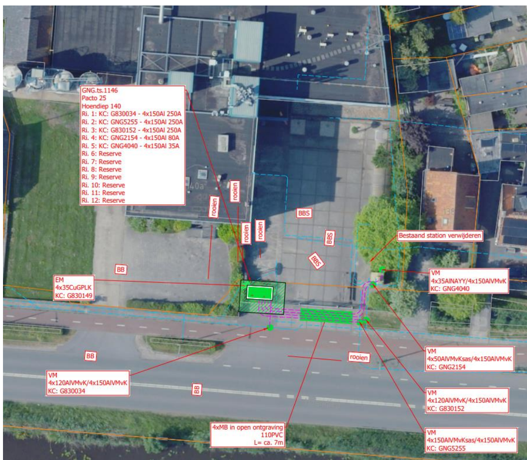
Figuur 1: De paarse stippellijn geeft de aan te leggen kabels aan binnen beperkingengebied II van een regionale waterkering.
