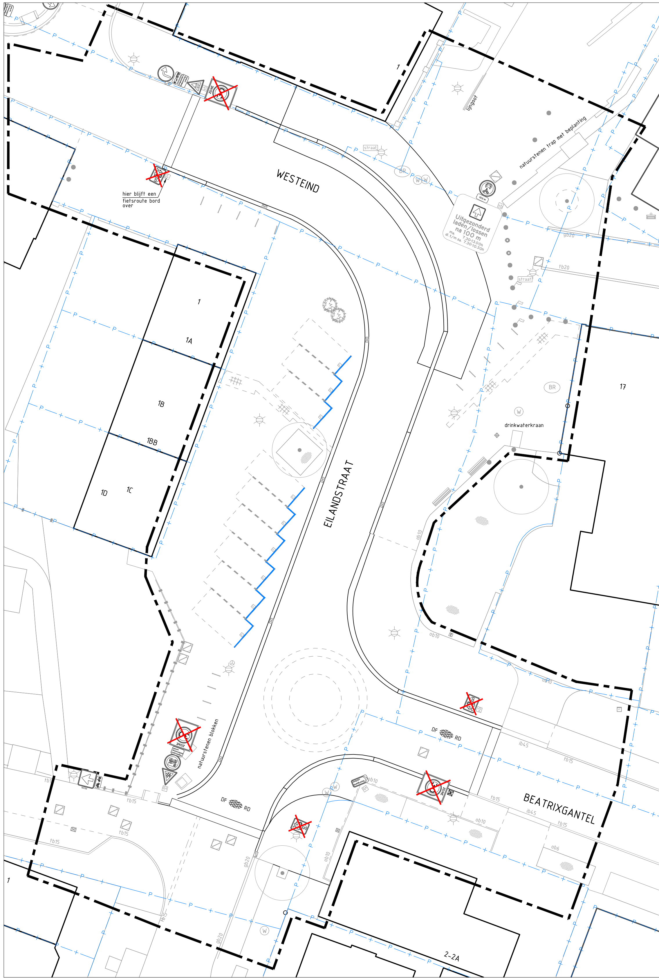
BESTAANDE SITUATIE INCL. OPBREEKWERK SCHAAL 1:200
