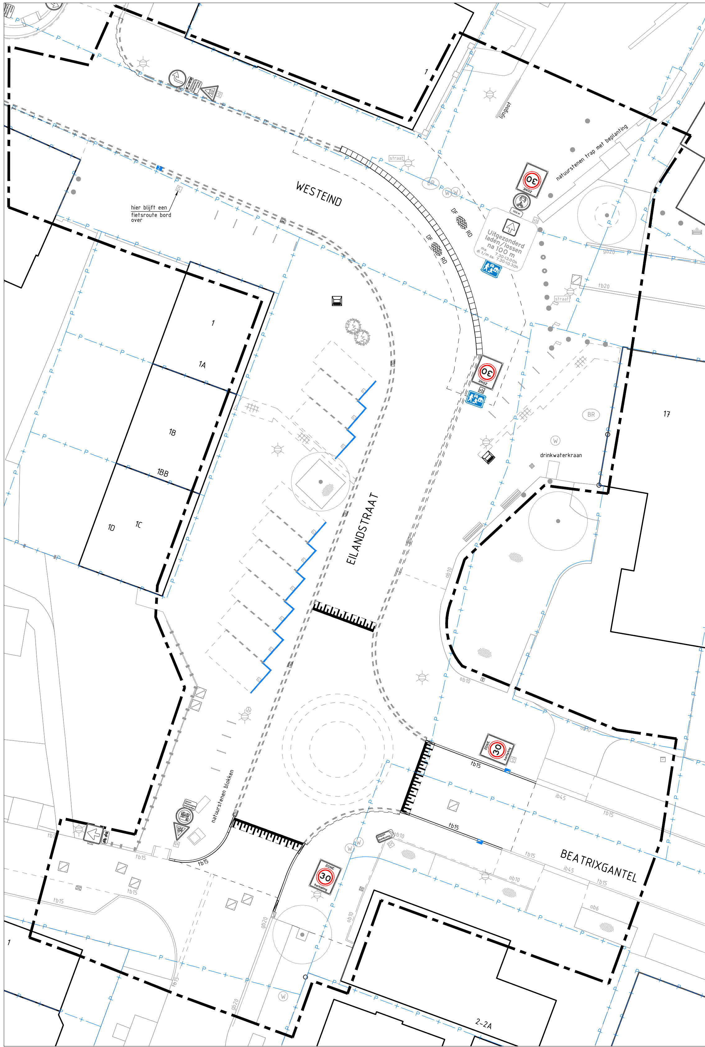
NIEUWE SITUATIE SCHAAL 1:200
