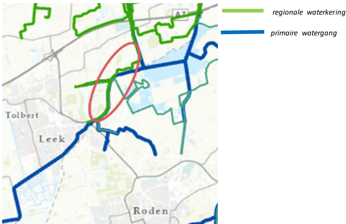
Figuur 1: globale aanduiding tracé fietspad
