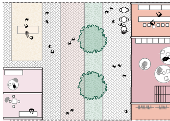
plattegrond wonen, woonentrees en programma aan de Levensader
