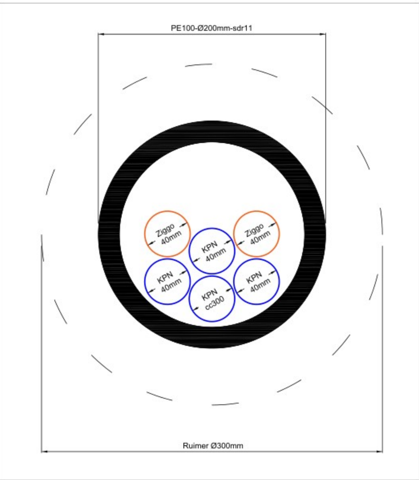
Dwarsdoorsnede buis (schaal 1:2)
