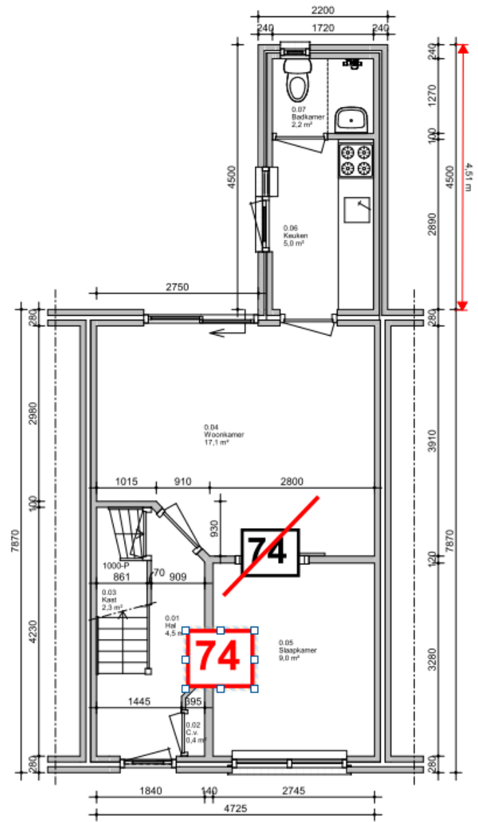
Begane grond Borneostraat
