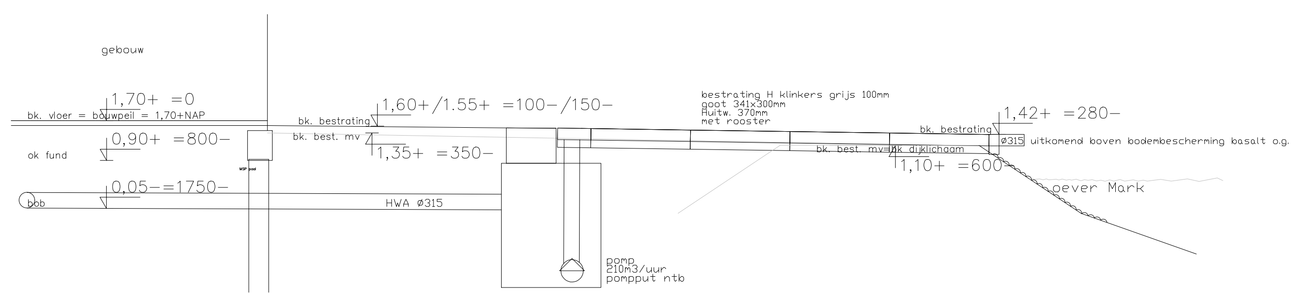
Doorsnede B-B
