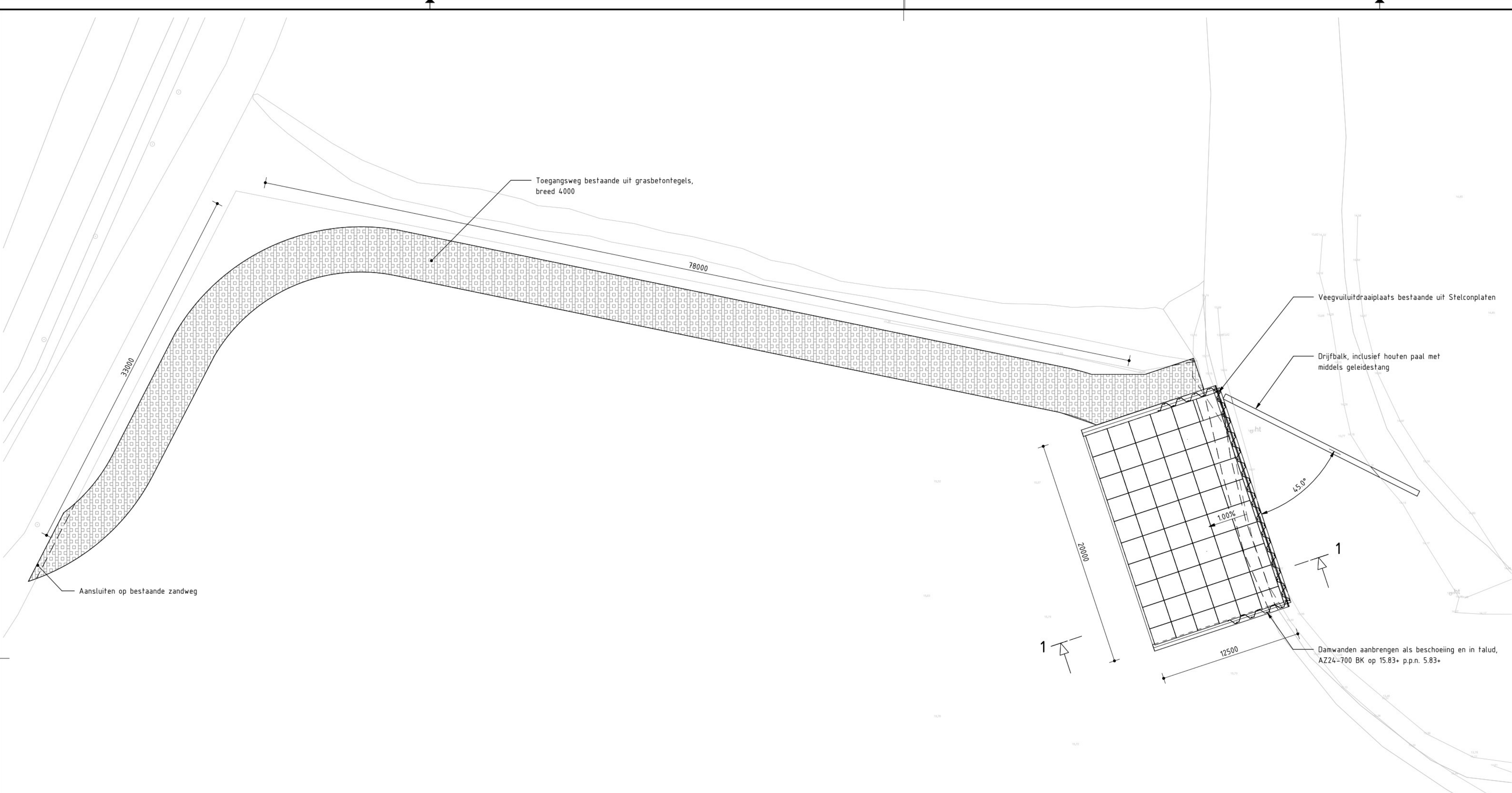
BOVENAANZICHT VEEGVULUITDRAAIPLAATS MET TOEGANGSWEG
