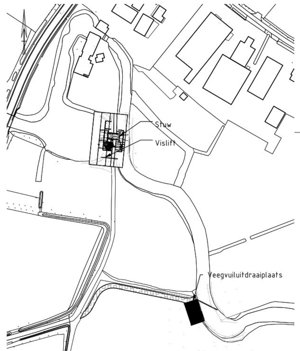
OVERZICHT CONSTRUCTIES NIEUW
