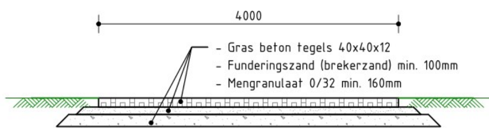
PRINCIPE DOORSNEDE TOEGANGSWEG
