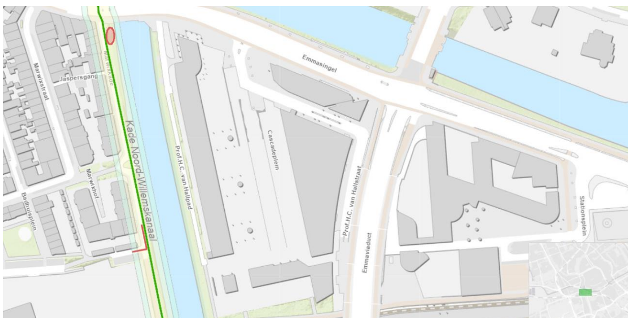
Figuur 1: De rode lijn geeft het aan te leggen leidingtracé aan binnen beperkingengebied I en II van een regionale waterkering waarvoor de vergunningplicht geldt. In de rode eclips wordt een gasstation met bijbehorende afsluiters en afblaas verwijderd uit beperkingengebied I van een regionale waterkering.
