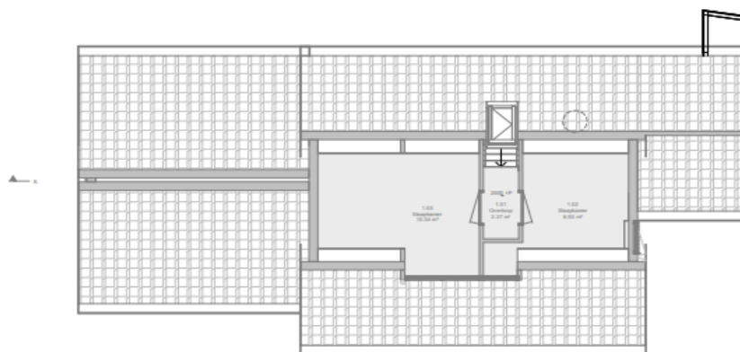
Bestaande 1e Verdieping
