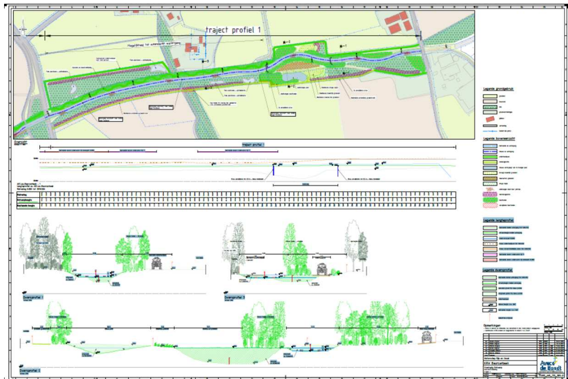
Figuur 2: Traject 1 van de herplantlocaties, gelegen ten noorden van de Beurzerbeek. Herplant vindt plaats aan de noordkant van de Beurzerbeek.
