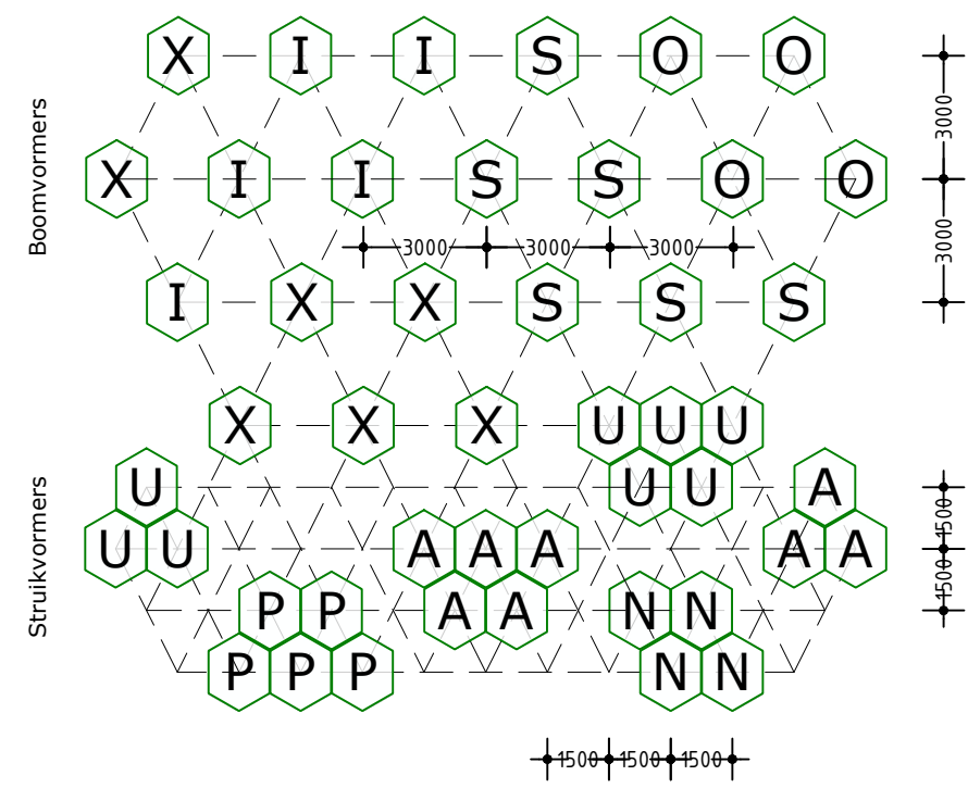
PLANTAFSTANDEN Schaal 1:200
