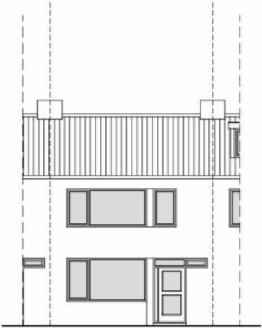
Voorgevel (Bestaande situatie)
