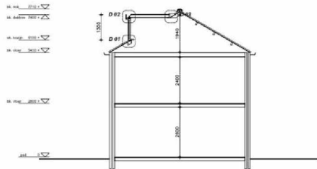
Doorsnede A-A (Nieuwe situatie)
