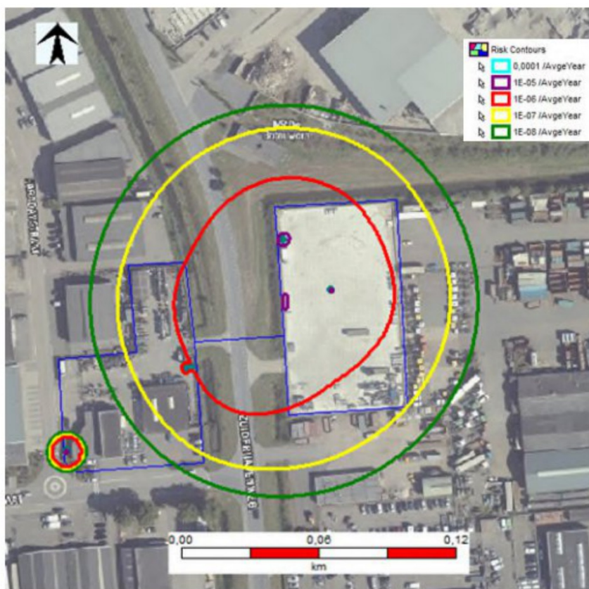
Figuur 2. Ligging PR 10^{-6} contour
