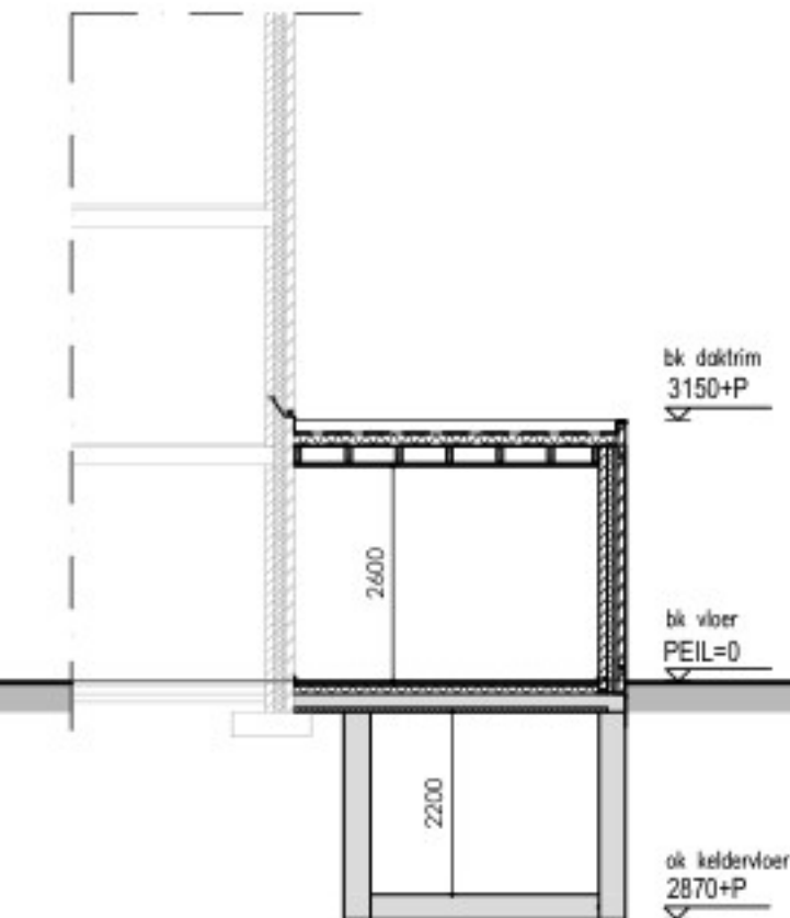
DOORSNEDE NIEUW
