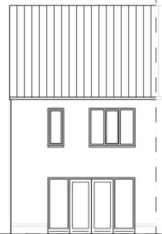
ACHTERGEVEL BESTAAND
