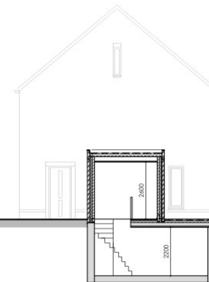
DOORSNEDE NIEUW
