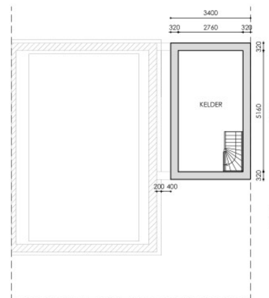
KELDER NIEUW
