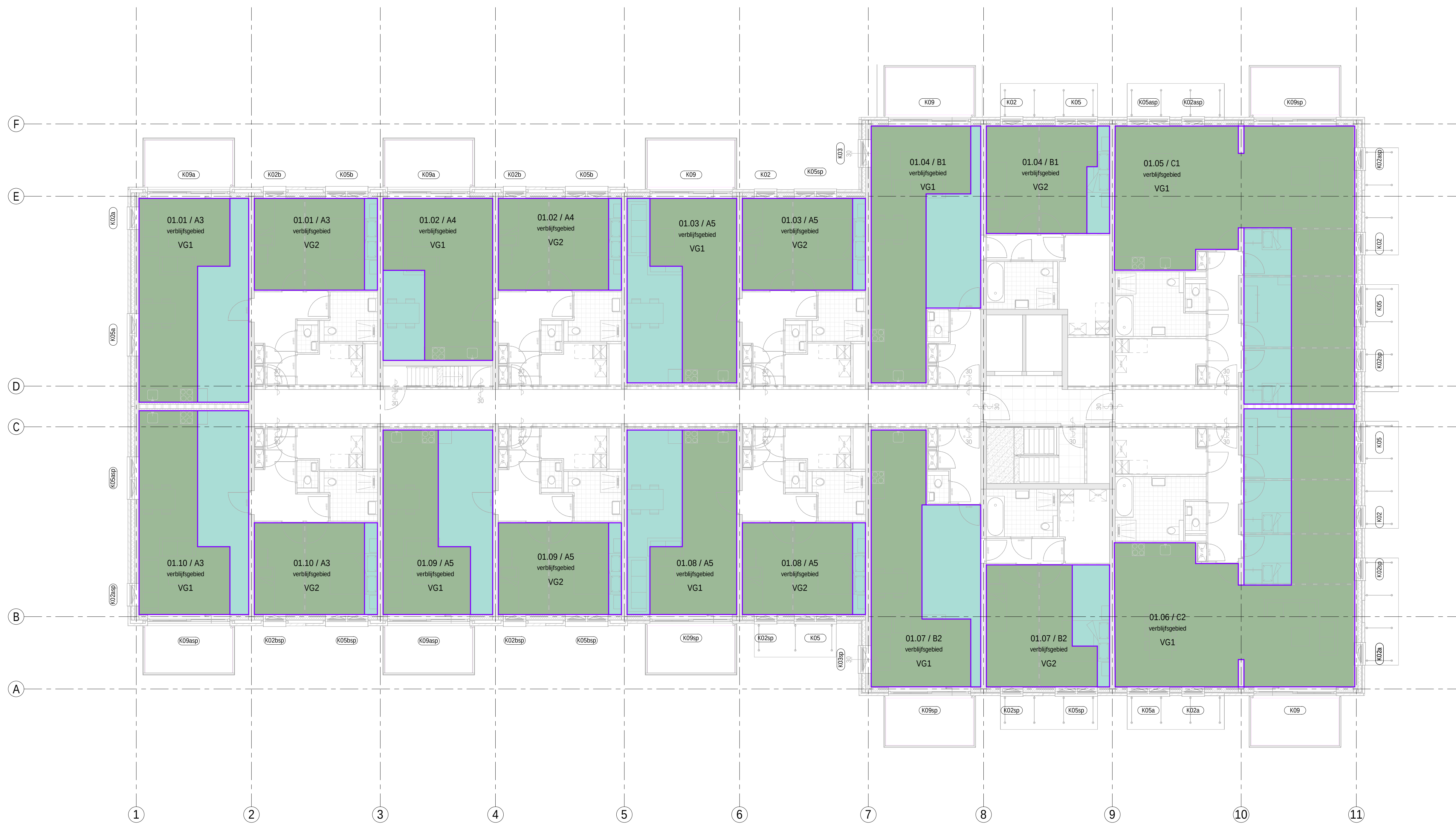
01 eerste verdieping
