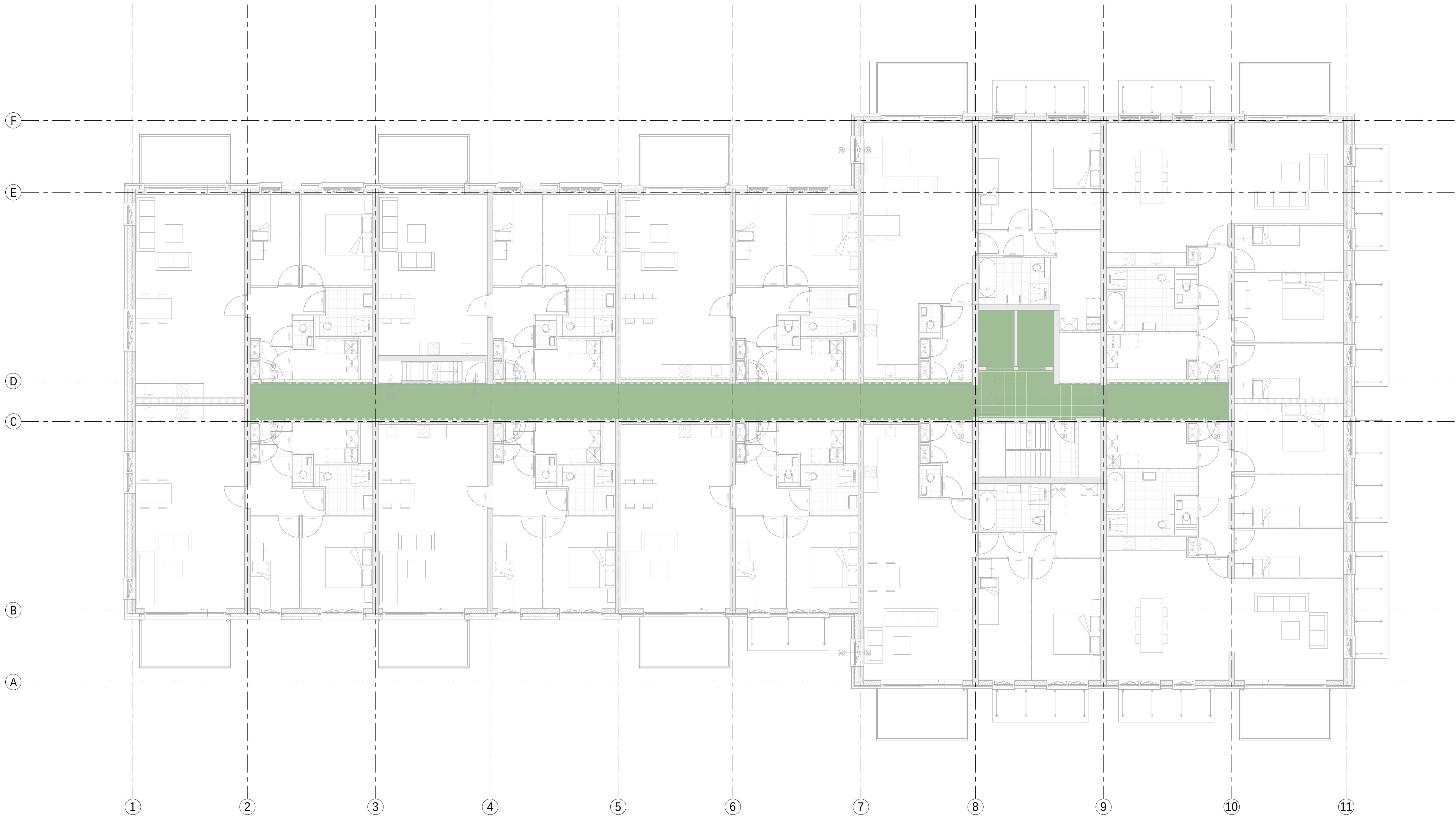
01 eerste verdieping
