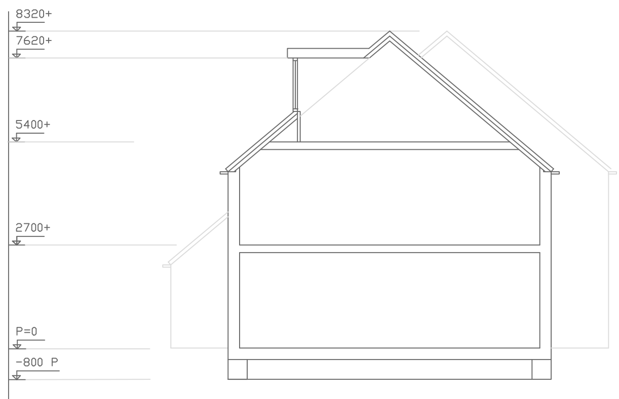
DOORSNEDE bestaand
