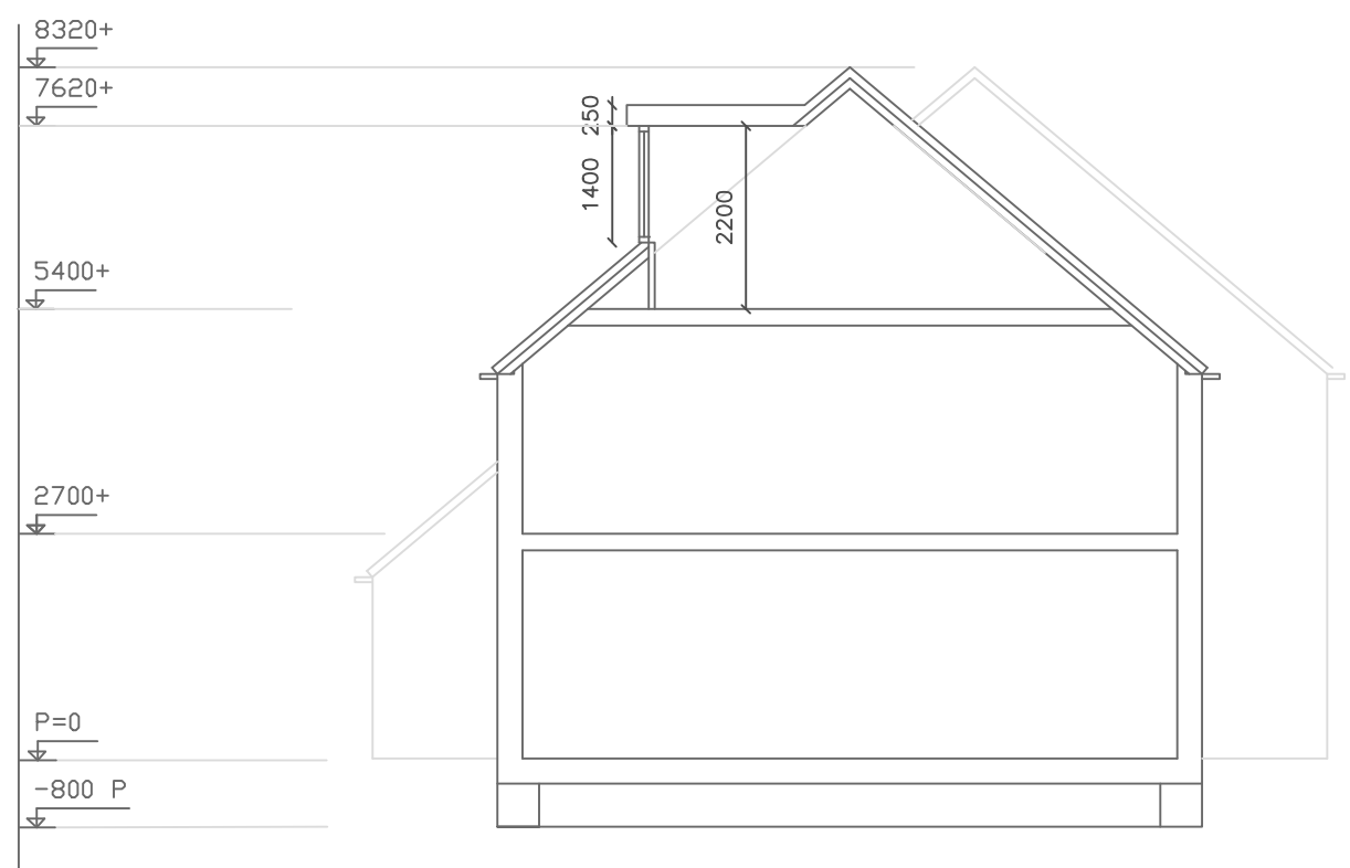
DOORSNEDE nieuw
