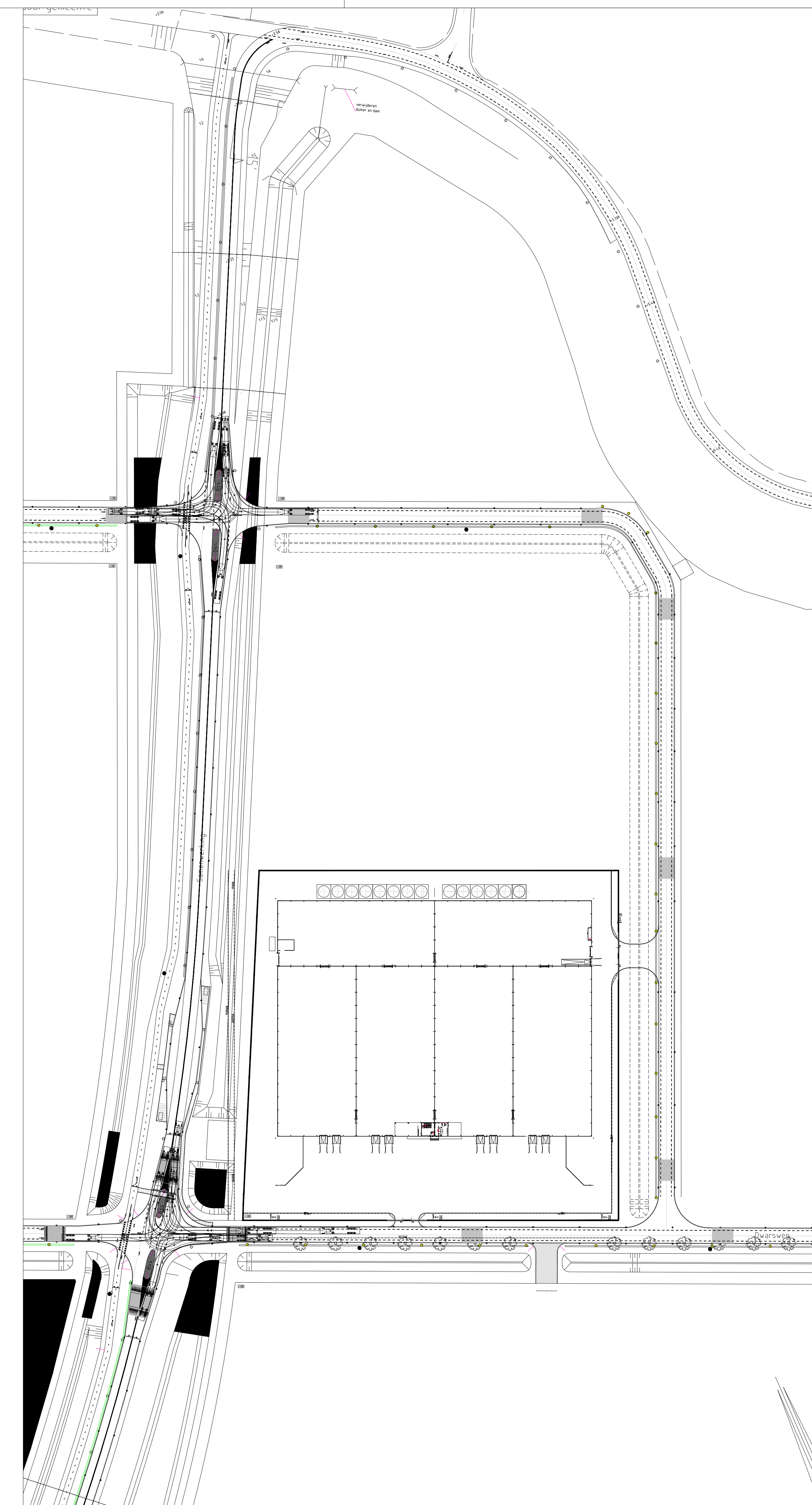
Situatie Bestaand 1:1000
