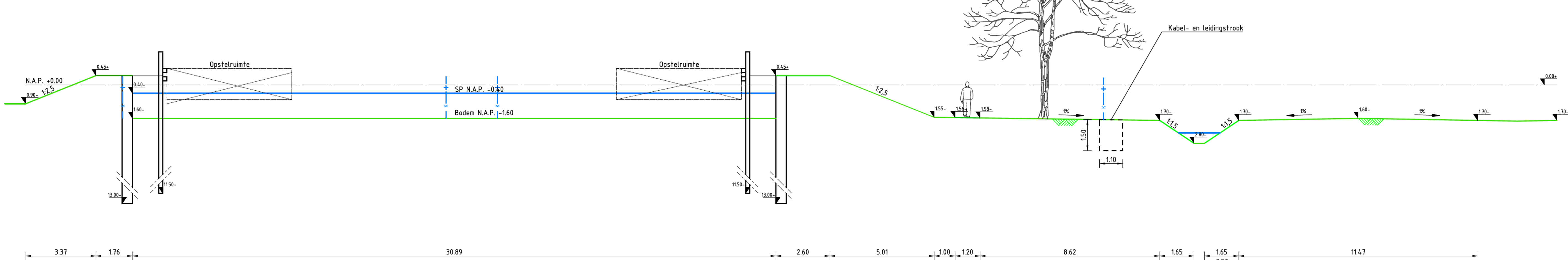
DOORSNEDE A SCHAAL 1 : 100
