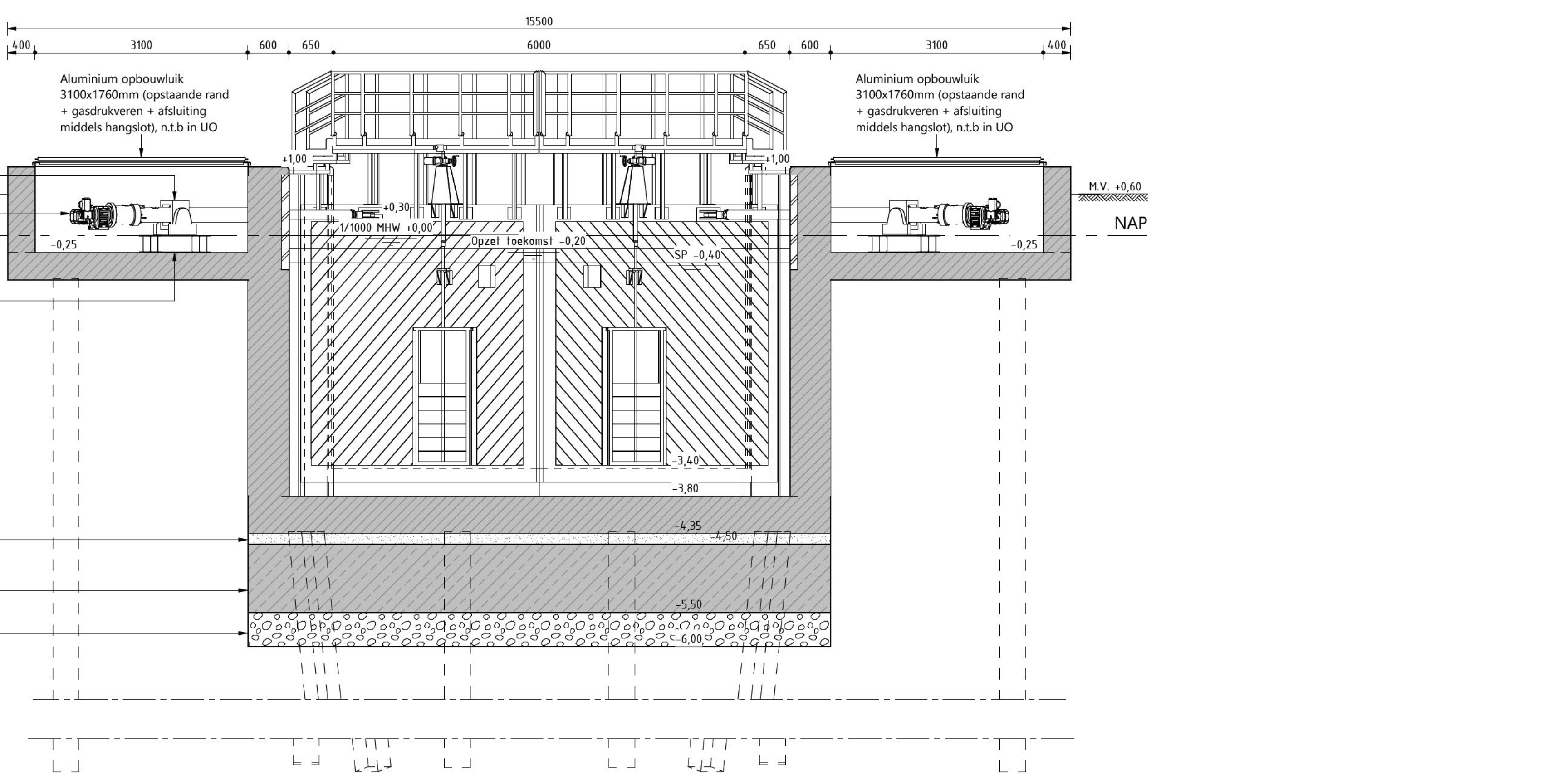
DWARSDOORSNEDE D-D BUITENHOOFD
