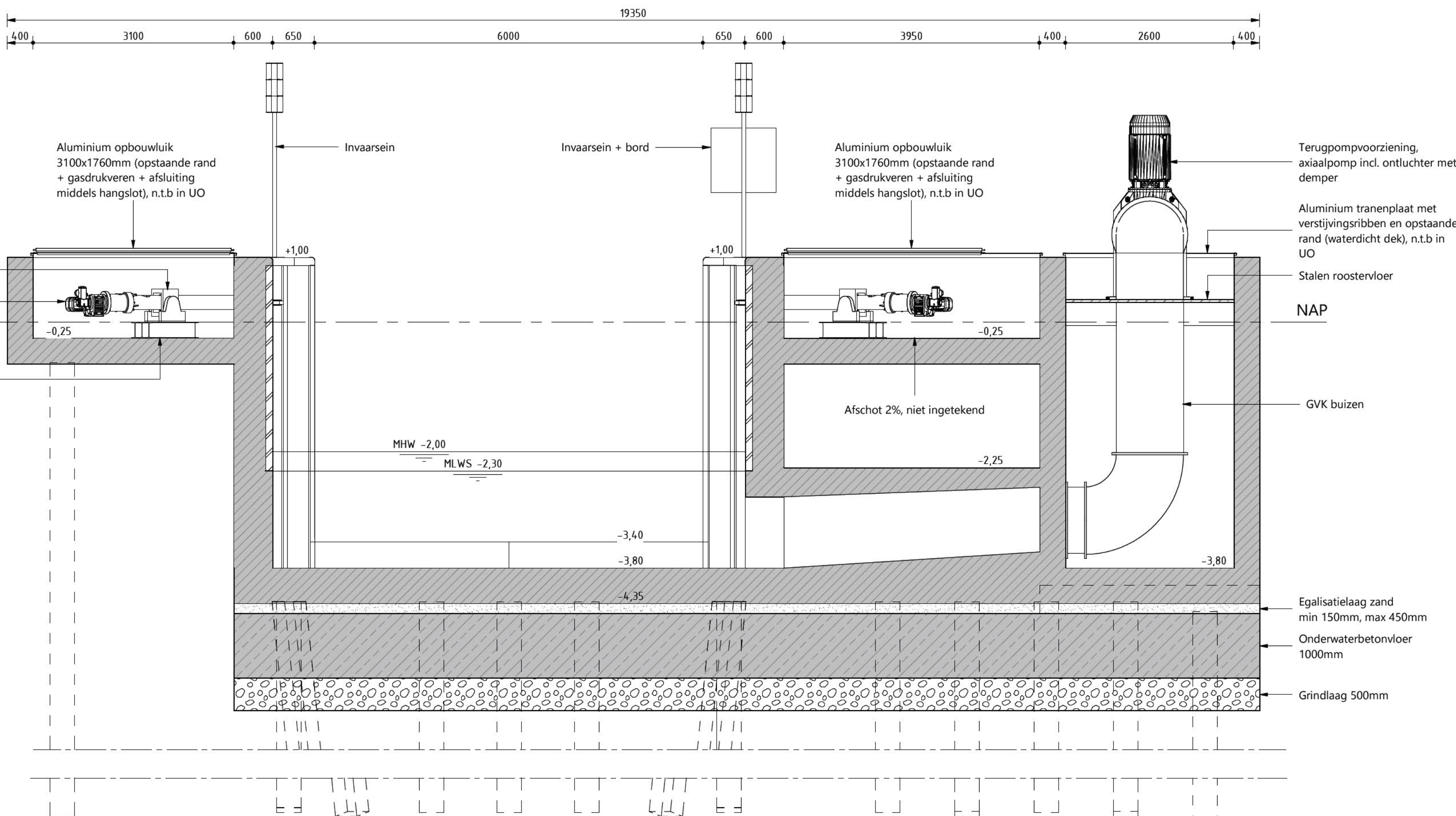
DWARSDOORSNEDE B-B BINNENHOOFD
