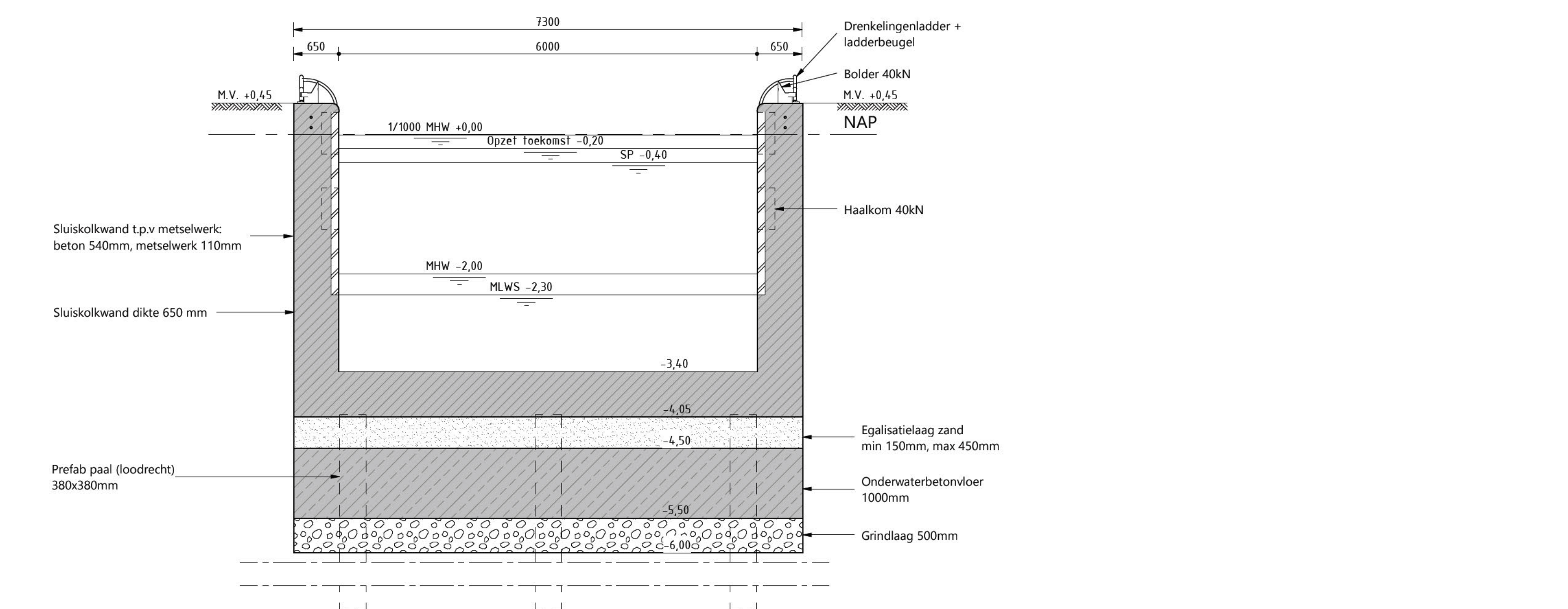
DWARSDOORSNEDE C-C KOLK
