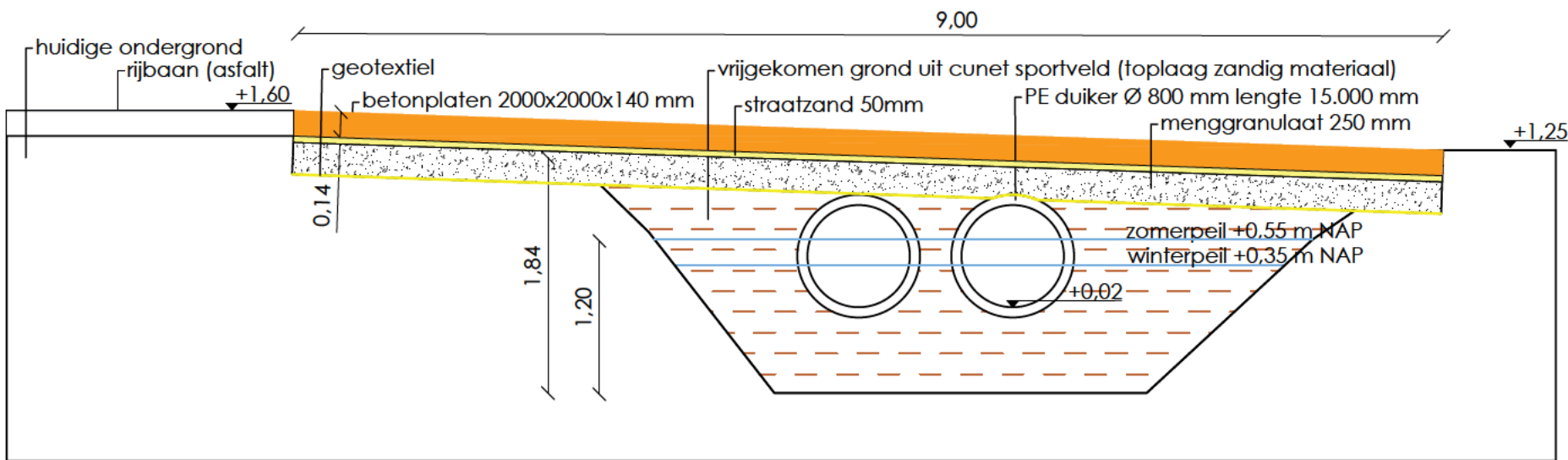
Principedetail dam met 2 duikers
